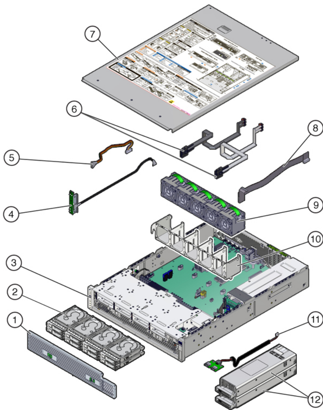
图 9 ZS5-2 存储、电源和风扇模块
