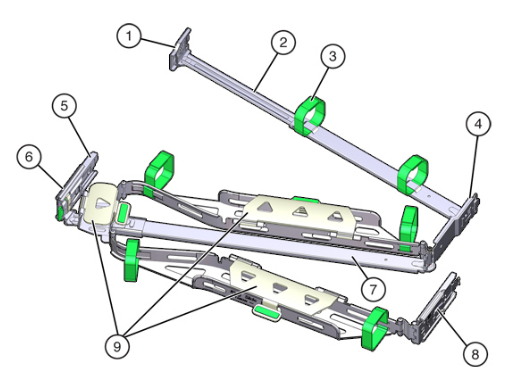
图 12 ZS5-2 控制器理线架
