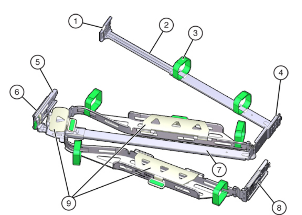
图 46 ZS3-2 控制器的可选理线架
