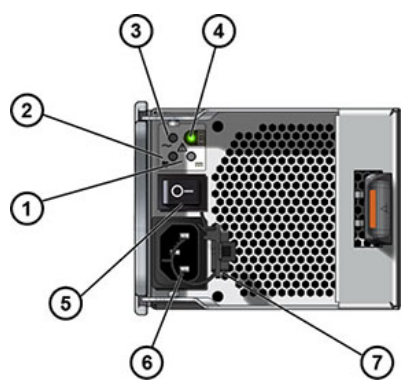
图 16 DE2 电源指示灯
