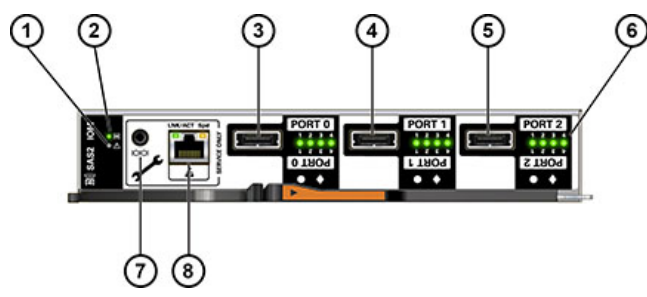
图 15 DE2 I/O 模块指示灯
