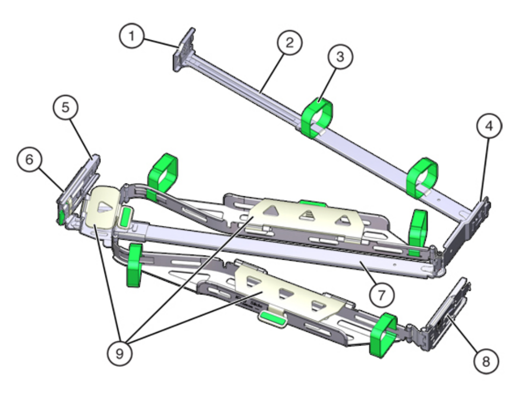
图 46 ZS3-2 控制器的可选理线架
