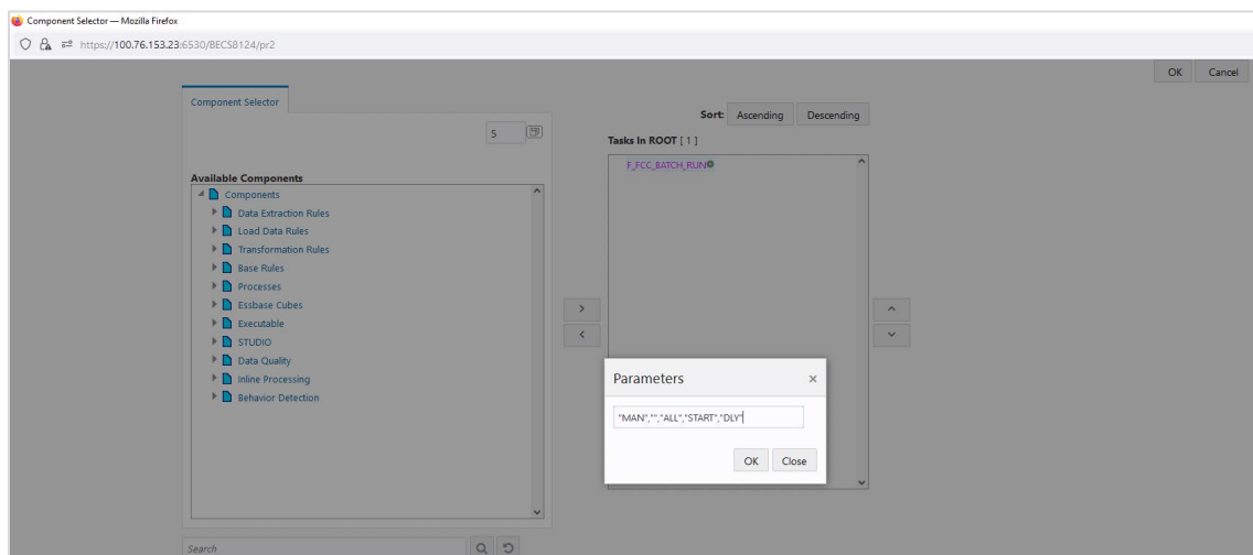
Figure 20: Parameters
