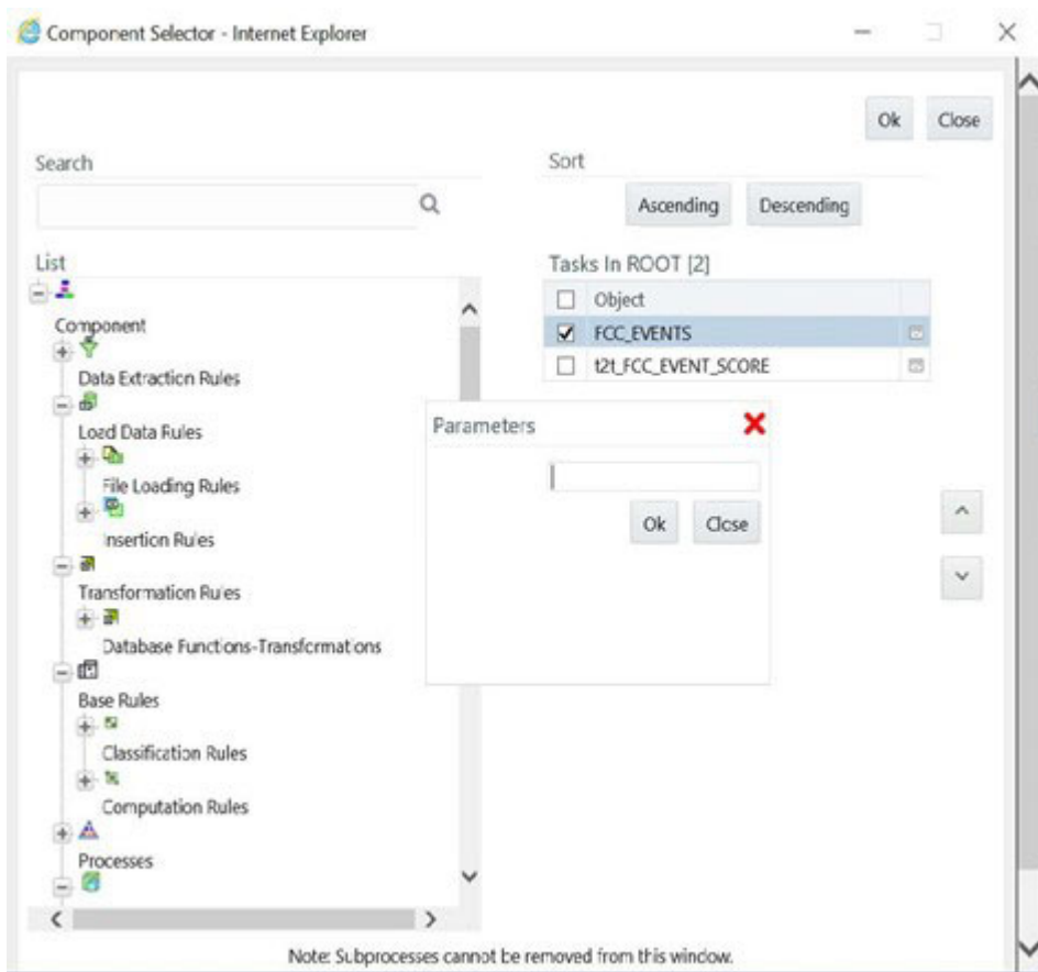
Figure 41: Parameters
