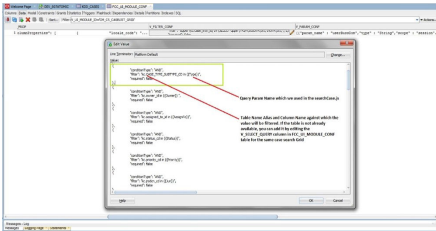
Figure 107: Parameters
