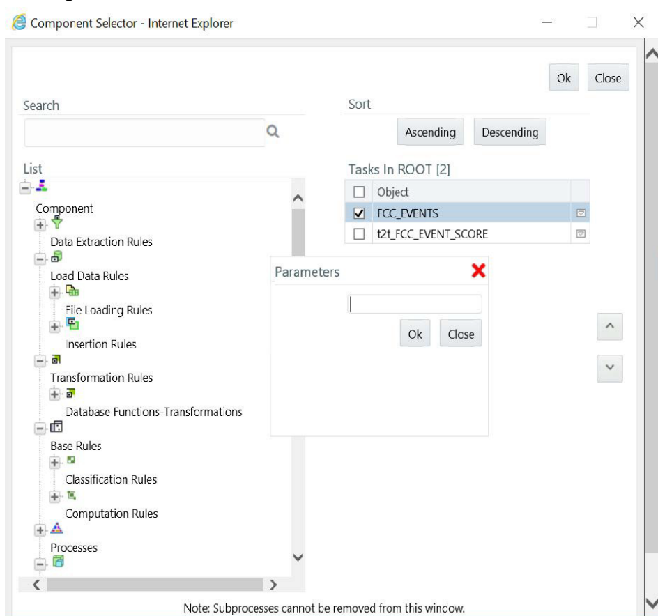
Figure 24: Parameters
