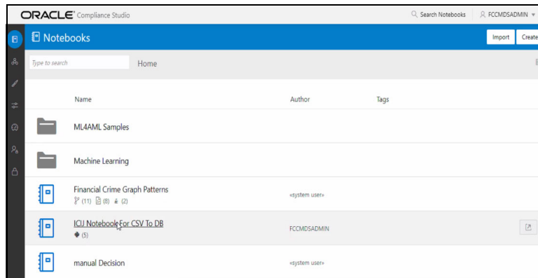
Figure 153: ICIJ Notebook
