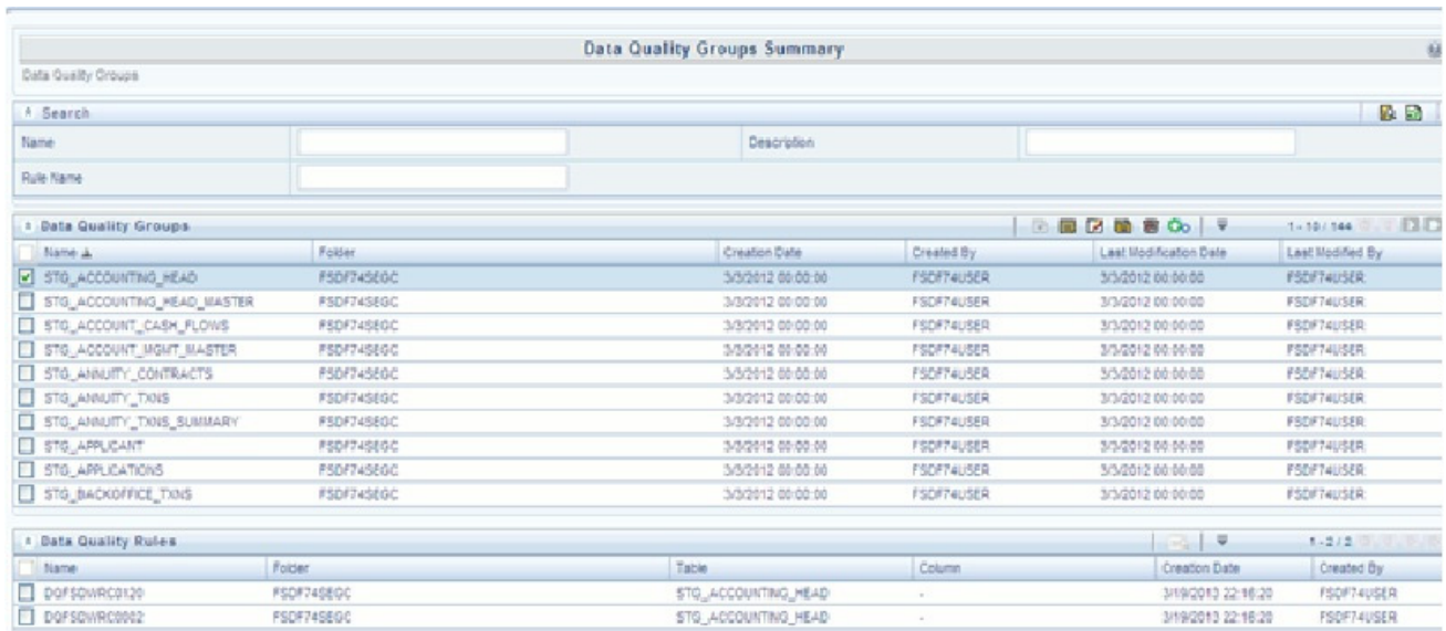
Figure 23. DQ Rules
