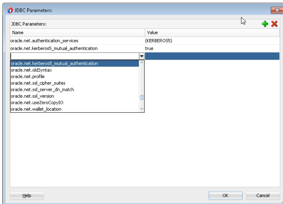
Figure 25-2 JDBC Parameters Dialog
