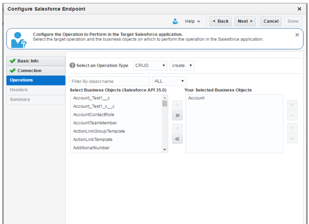
図 6-58 「操作」ページ
