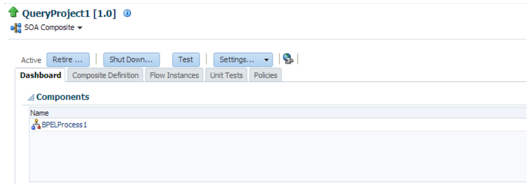
図 10-54 「テスト」タブ
