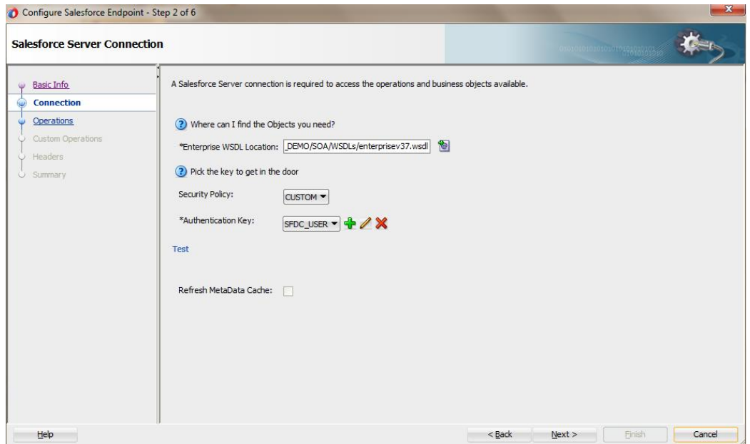
図 8-1 WSDL の場所
