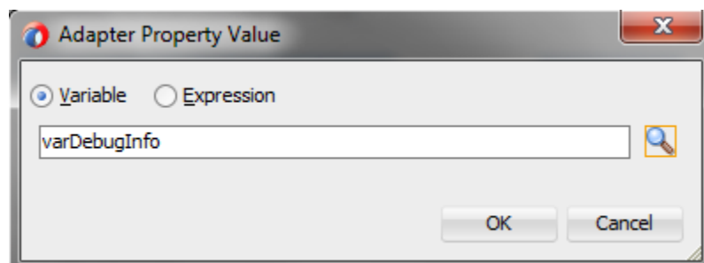
図 10-107 変数の選択
