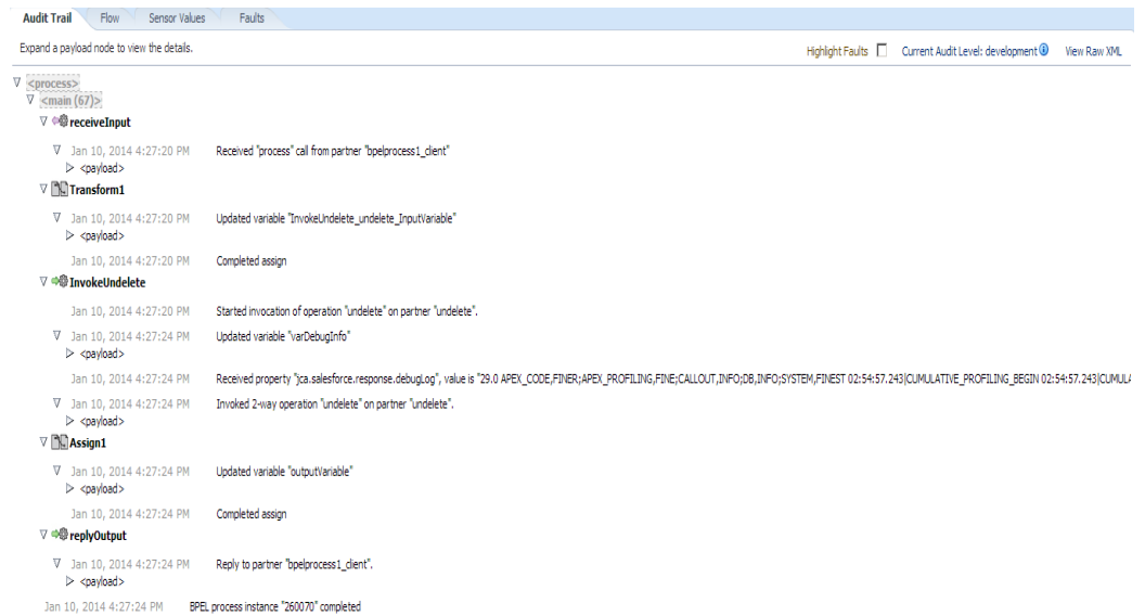
図 10-121 監査証跡
