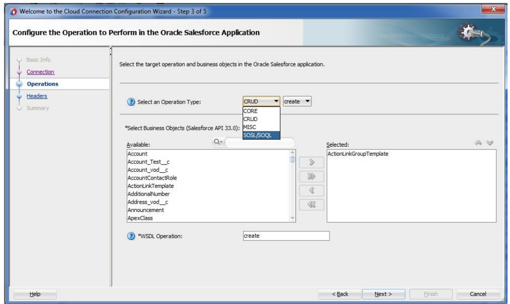
図 10-16 SOQL の選択
