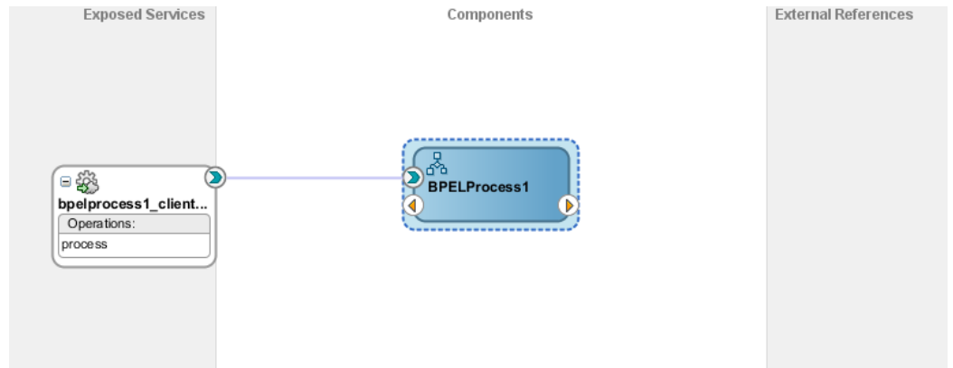
図 10-4 Composite.xml
