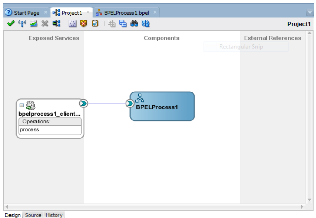
図 5-7 Composite.xml
