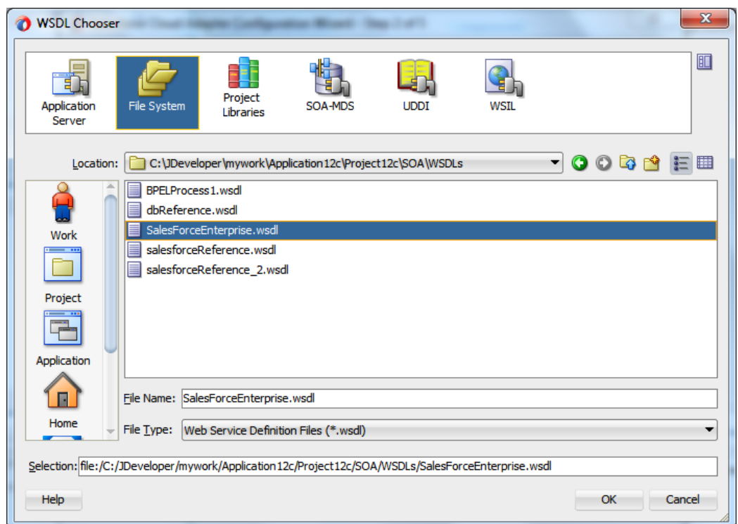
図 2-19 WSDL の選択
