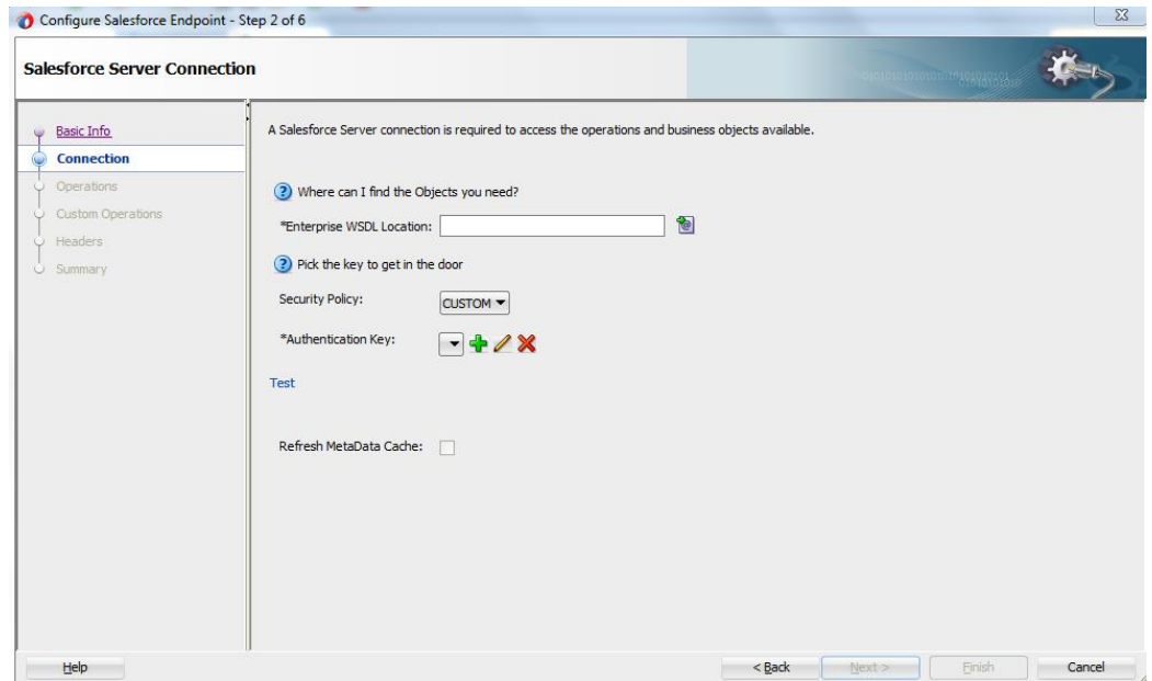
図 5-18 WSDL の場所
