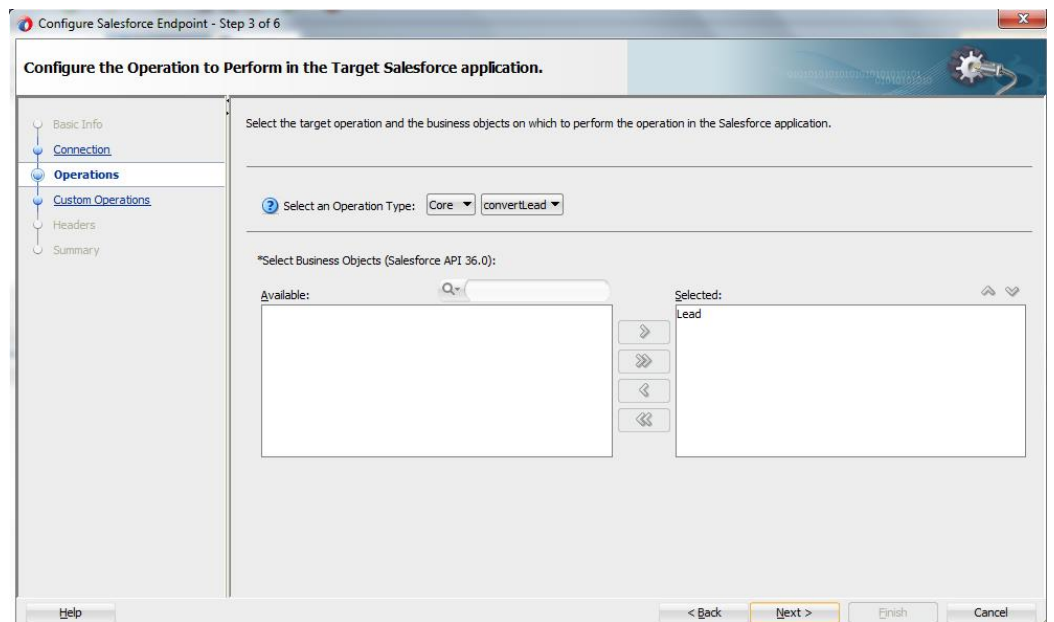
図 10-91 CORE の選択
