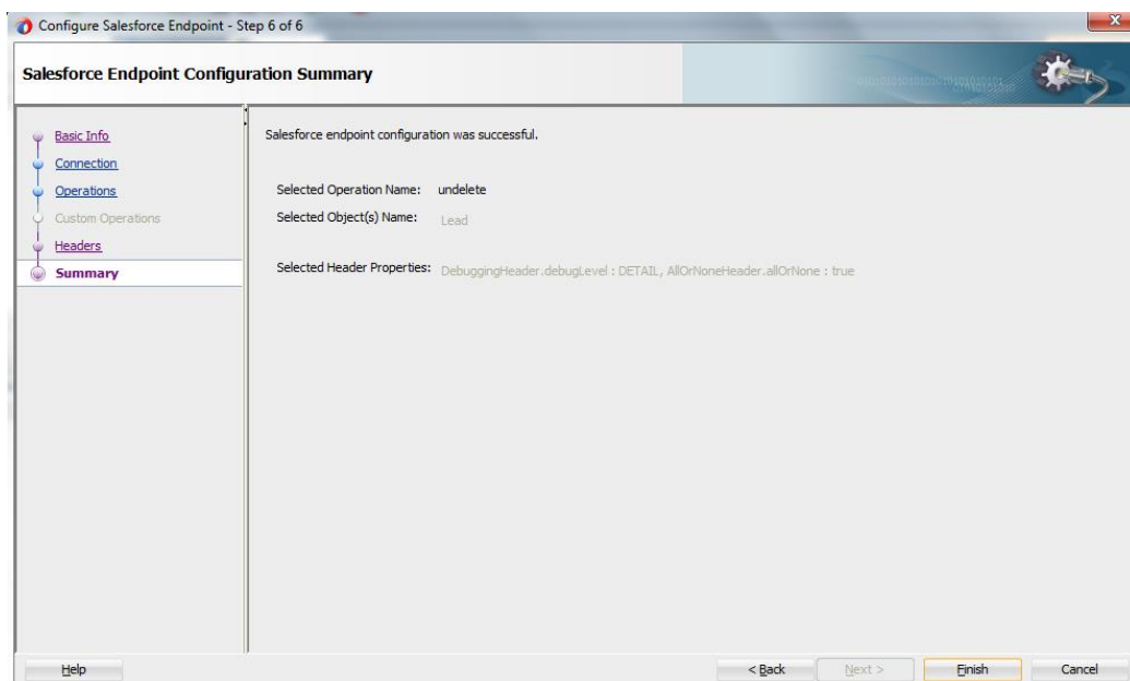
図 10-95 「終了」ページ
