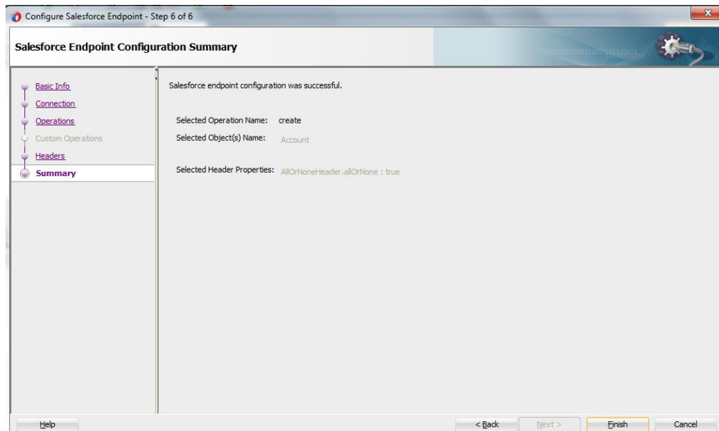
図 6-31 「終了」ページ
