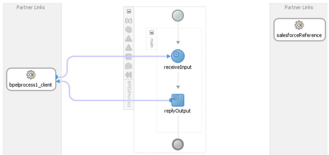
図 5-29 BPELProcess1 を開く
