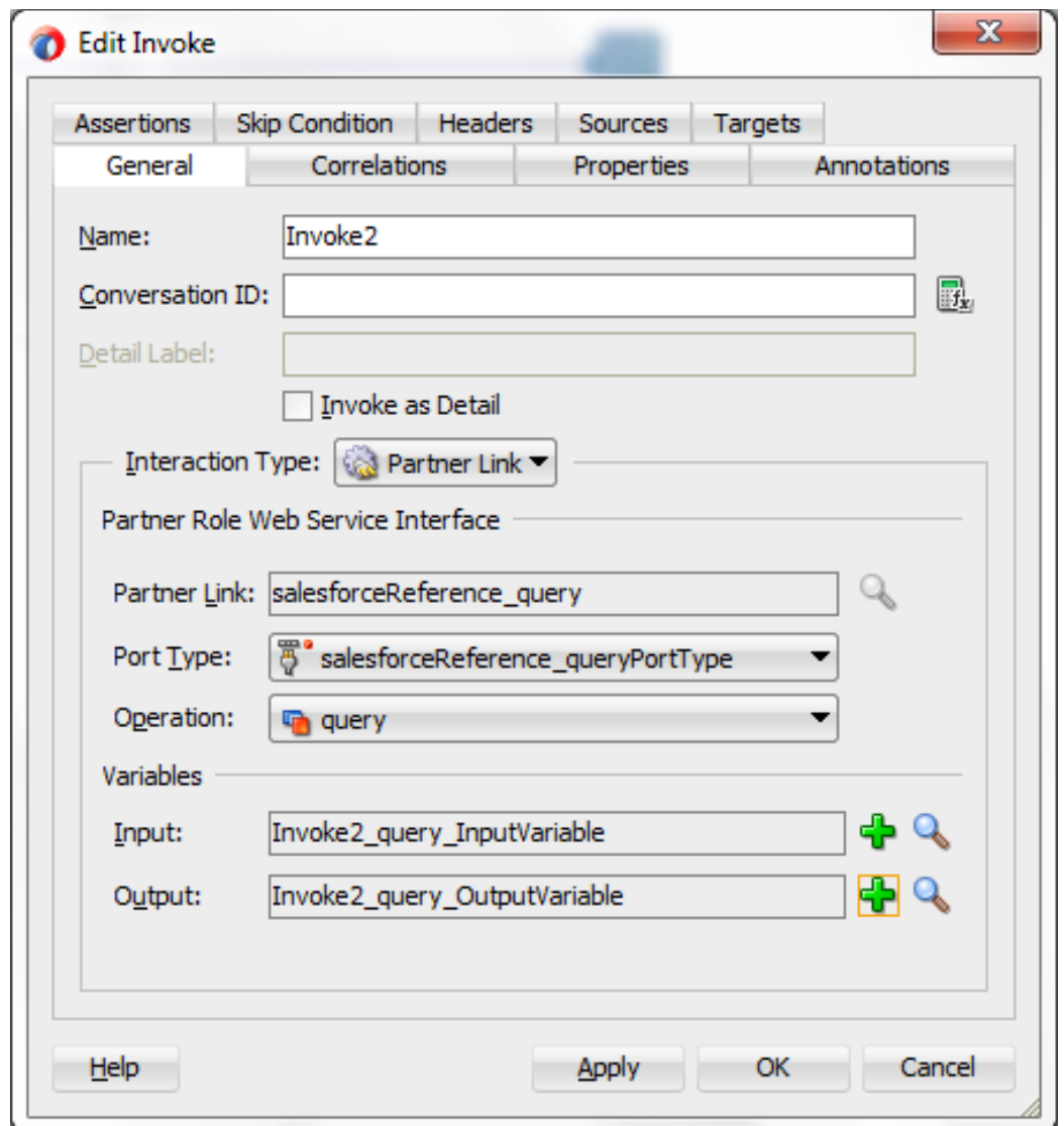
図 10-40 Invoke の編集
