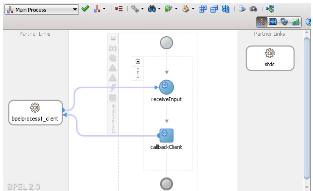
図 10-99 BPELProcess1 を開く
