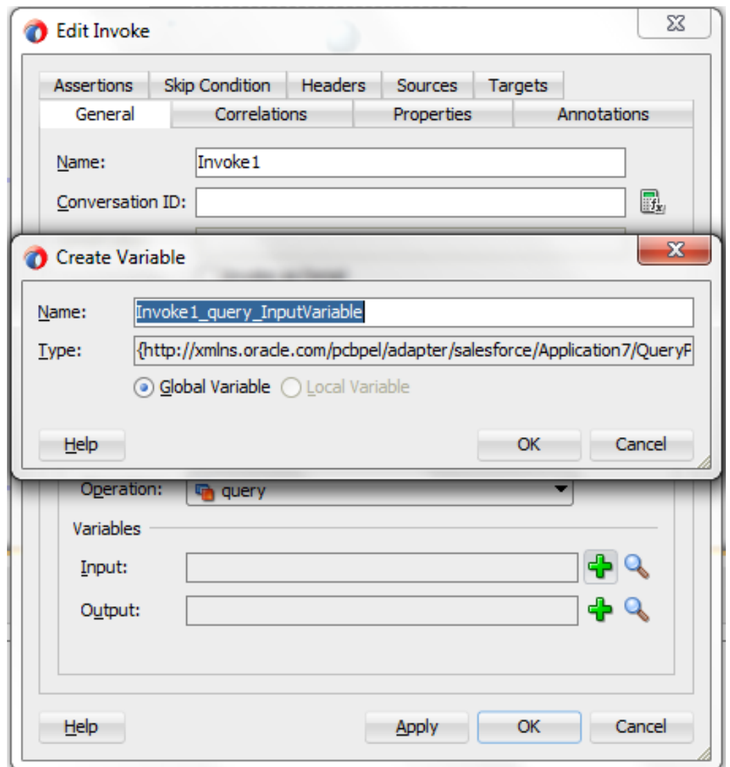
図 10-29 変数の作成
