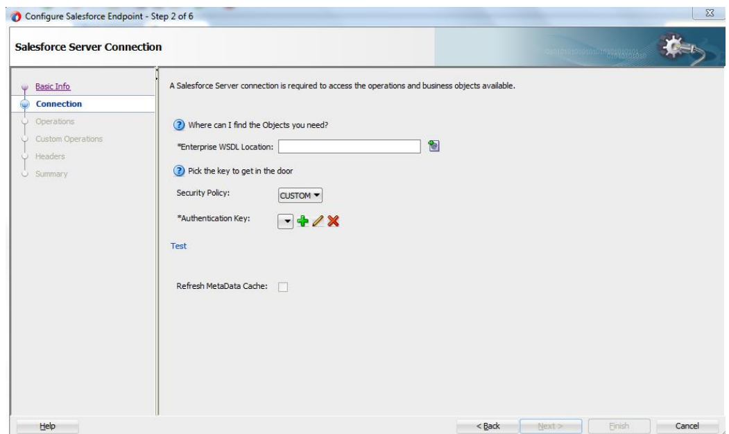
図 6-21 「接続」ページ
