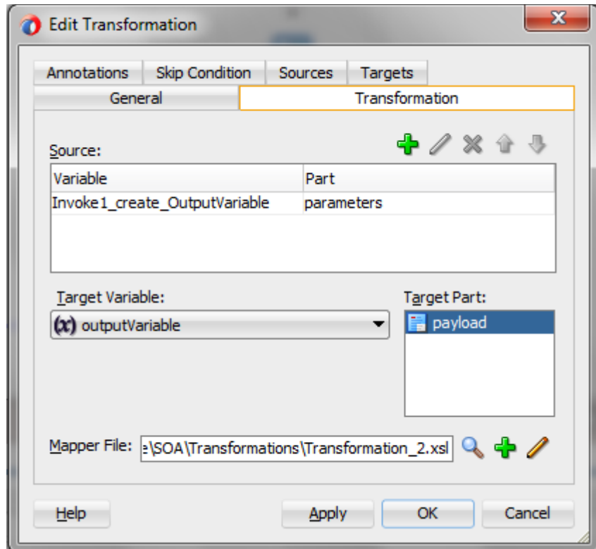
図 5-37 変換の編集
