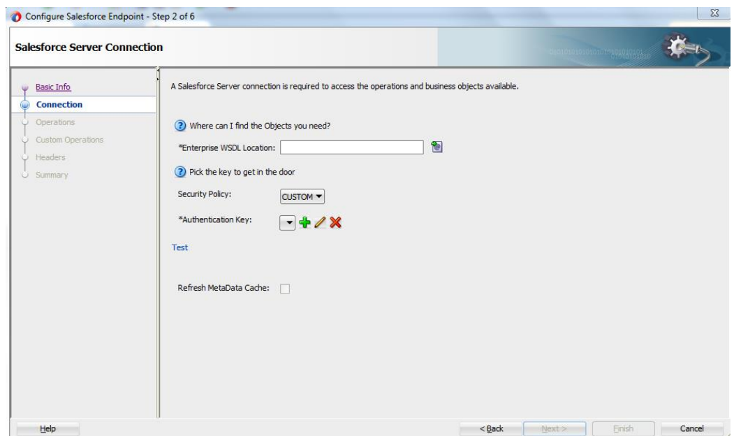
図 10-86 WSDL の場所
