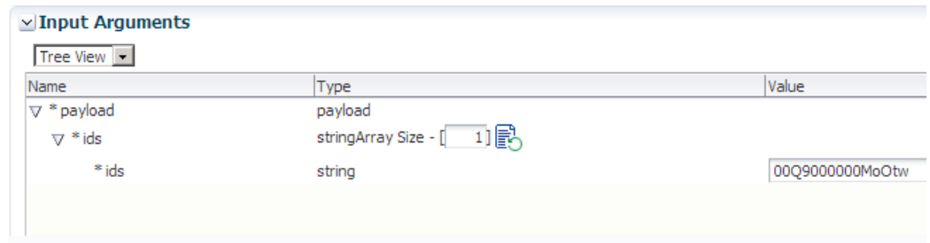
図 10-117 ID の入力
