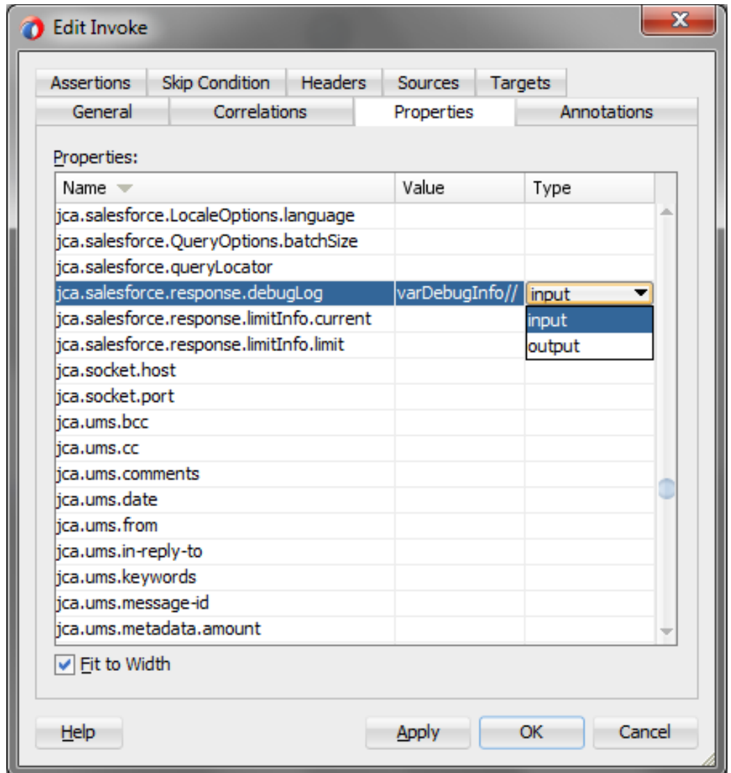
図 10-108 出力の選択
