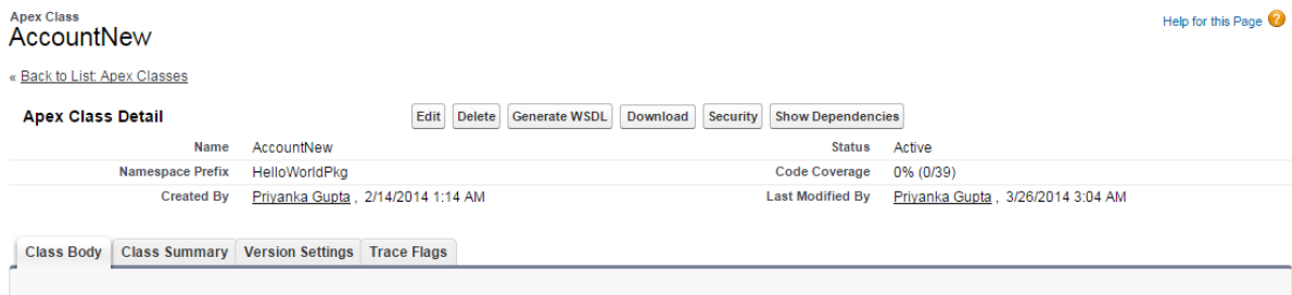
図 4-18 AccountNew
