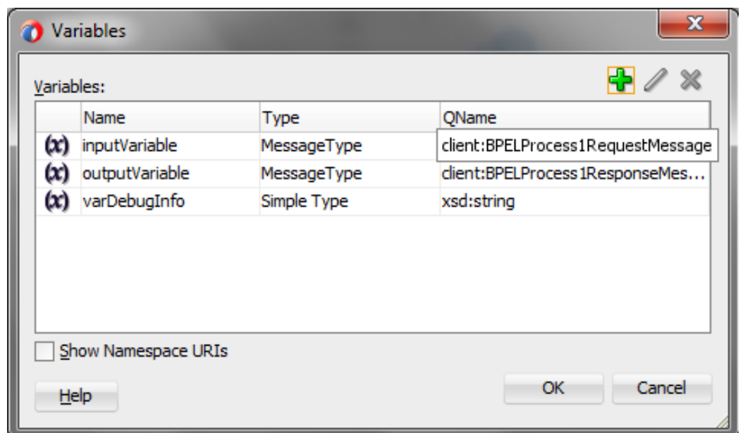
図 10-100 「変数」画面
