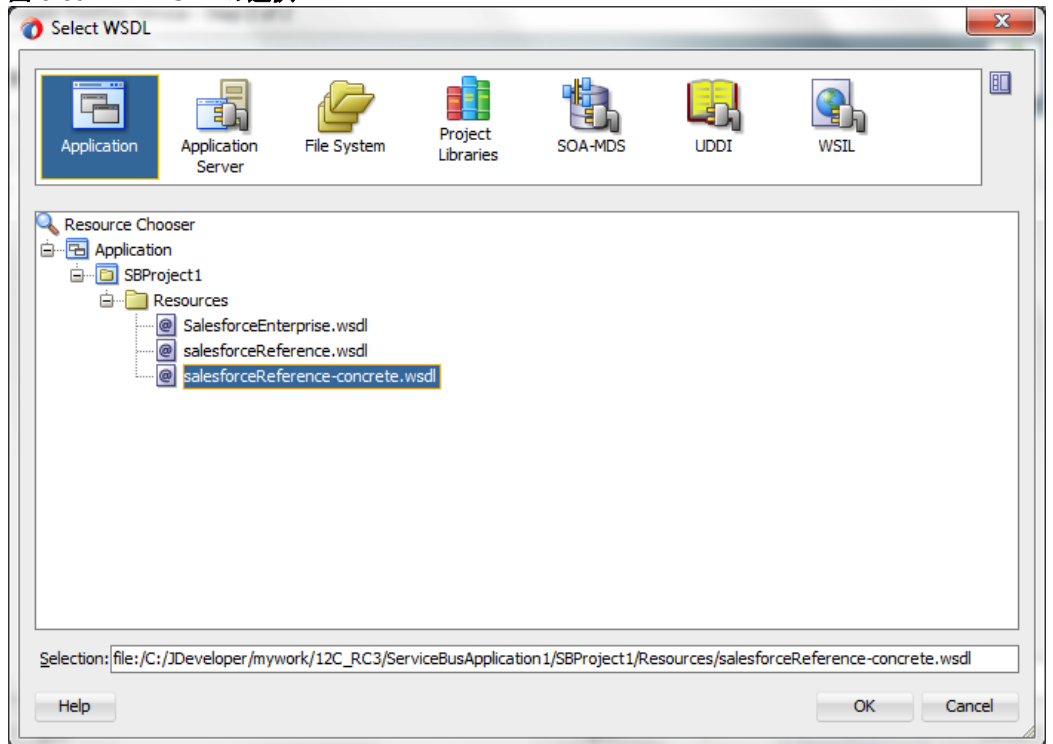
図 6-35 WSDL の選択
