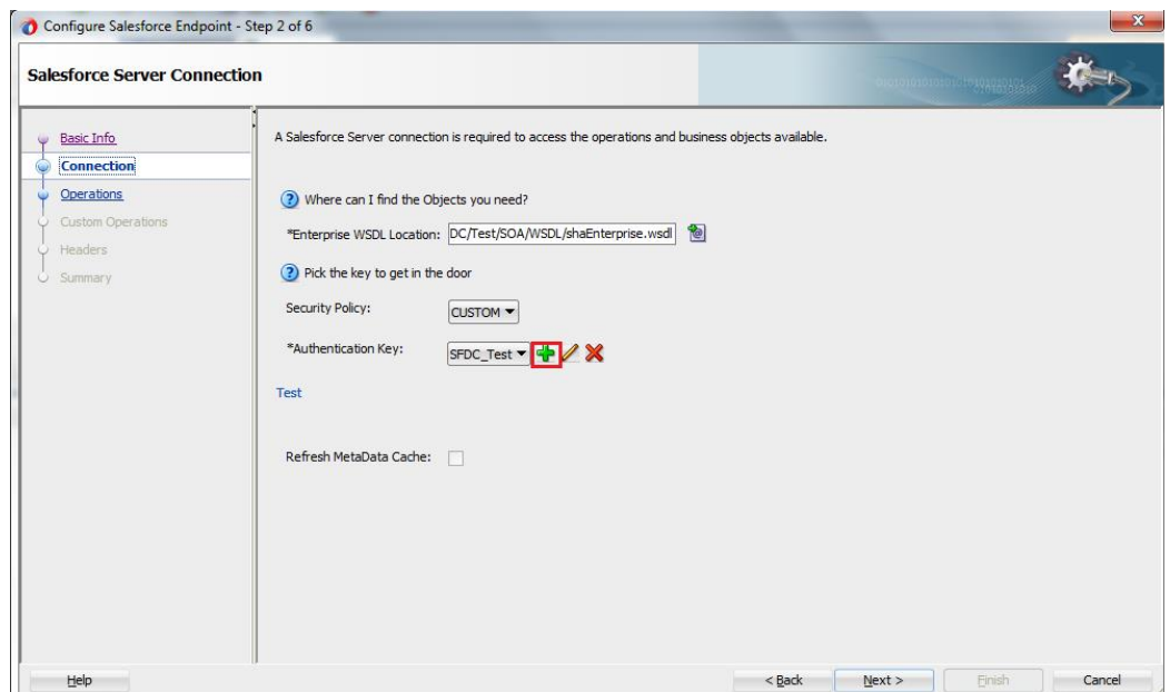
図 6-25 「接続」ページ
