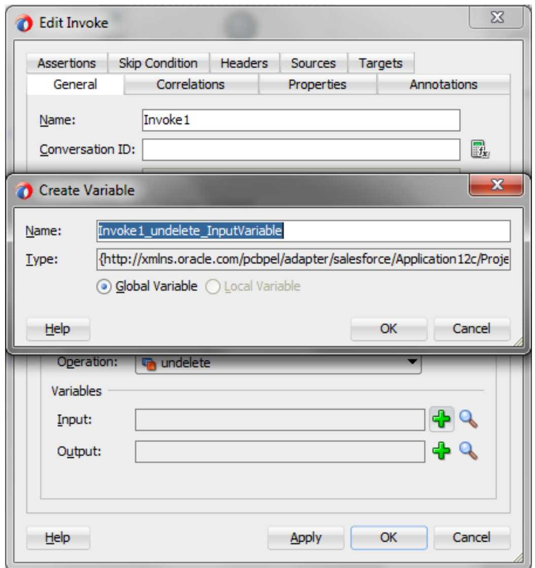
図 10-102 変数の作成
