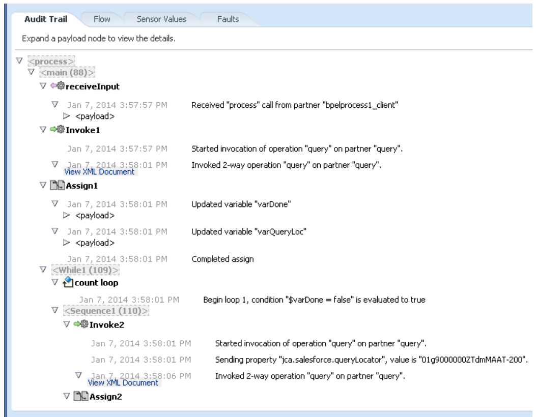
図 10-58 監査証跡
