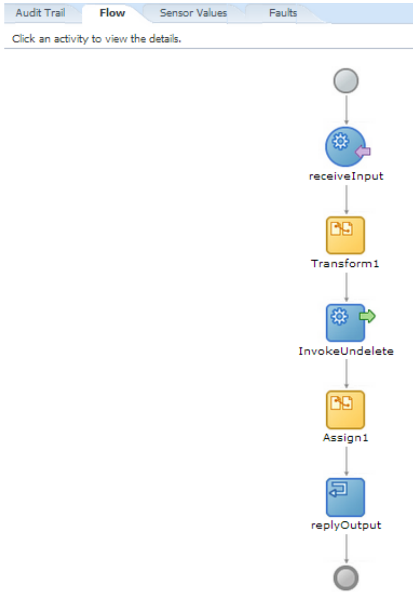
図 10-122 「フロー」タブ
