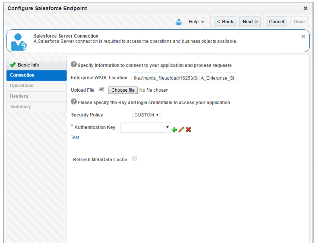
図 6-55 「接続」ページ
