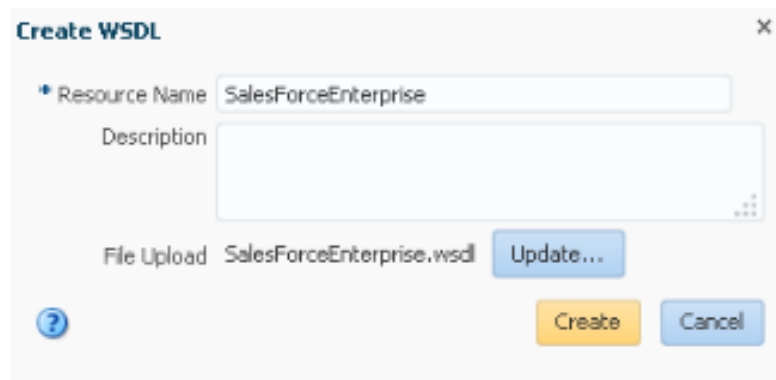
図 6-5 WSDL の作成
