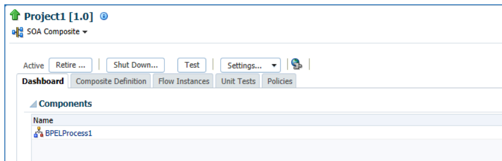
図 10-116 「テスト」タブ
