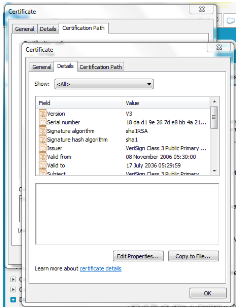
図 2-7 「Details」タブ
