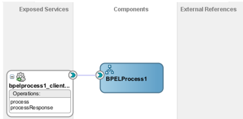
図 10-80 Composite.xml
