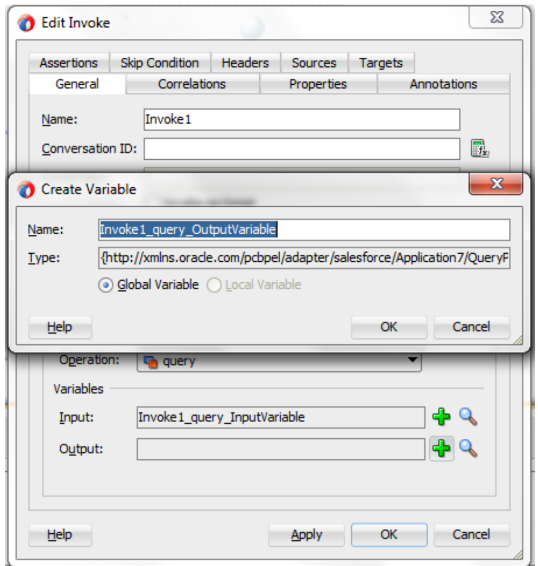
図 10-30 変数の作成
