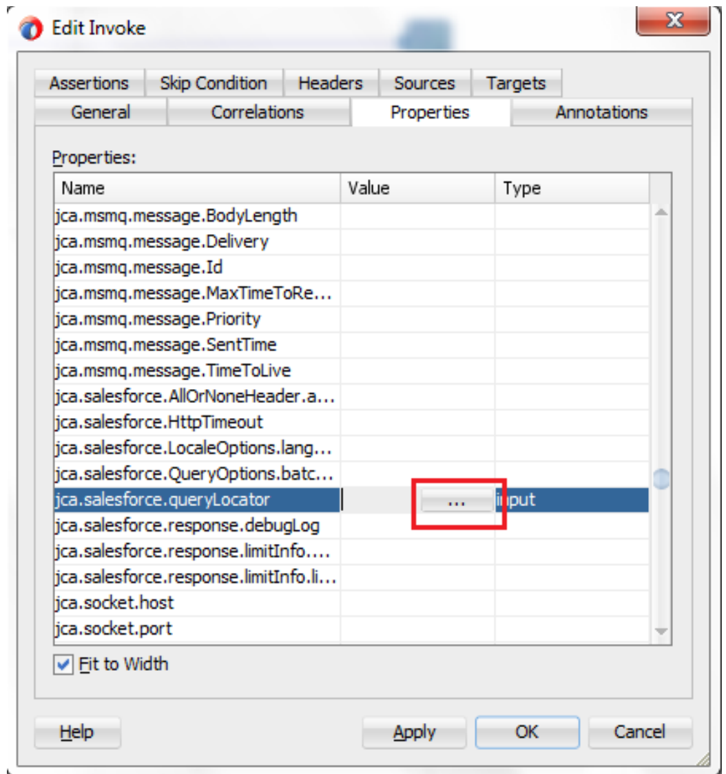
図 10-42 変数の参照
