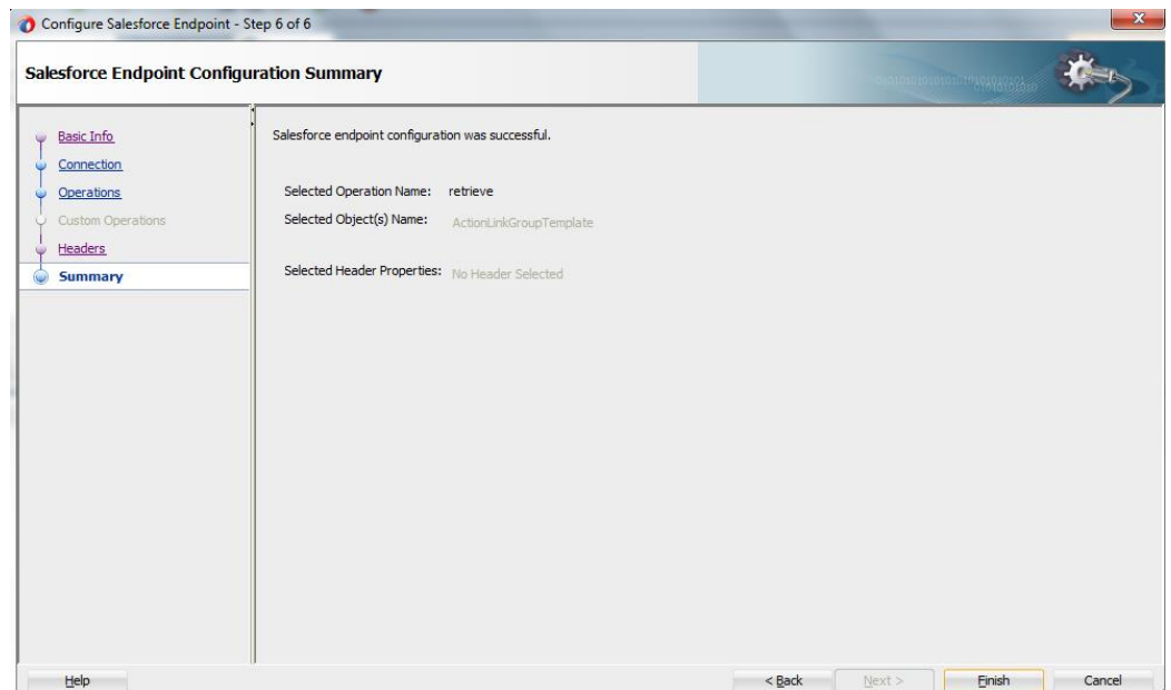
図 10-21 「終了」ページ
