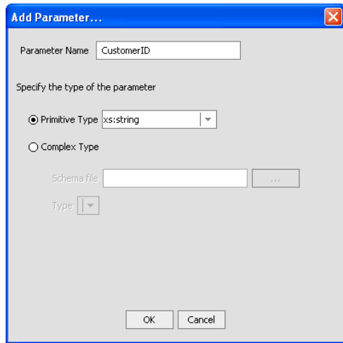
Figure 4-10 Add Parameter
