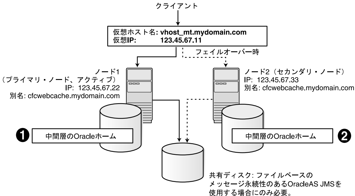
図 11-6 個別の Oracle ホームを使用した OracleAS Cold Failover Cluster (中間層) 構成
