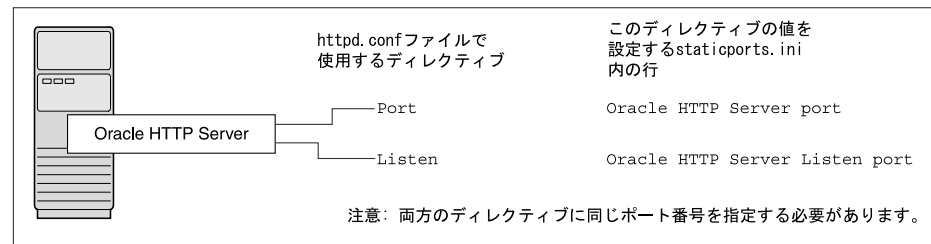
図 3-2 Oracle HTTP Server のみを構成する場合
