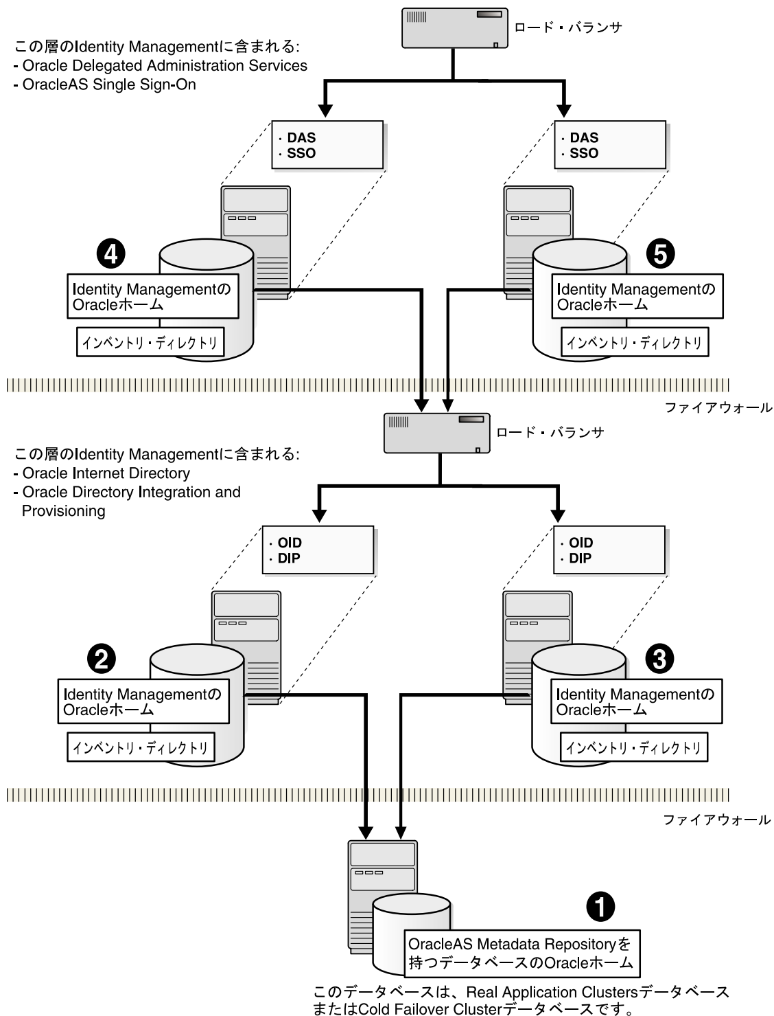
図 12-2 分散 OracleAS Cluster (Identity Management) 構成
