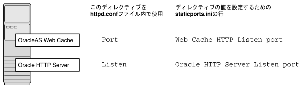
図 4-1 OracleAS Web Cache と Oracle HTTP Server の両方の構成
