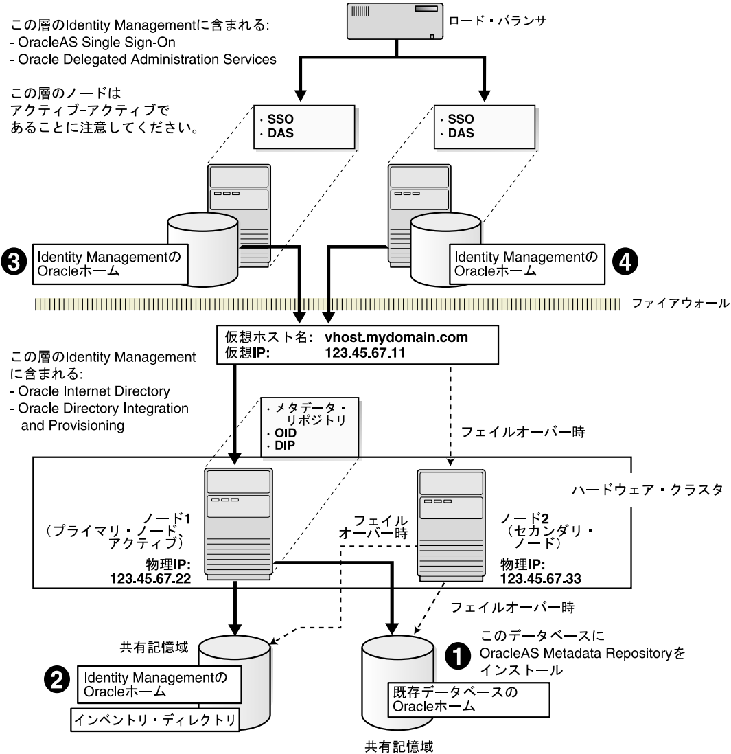
図 11-4 分散 OracleAS Cold Failover Cluster (Oracle Identity Management) 構成
