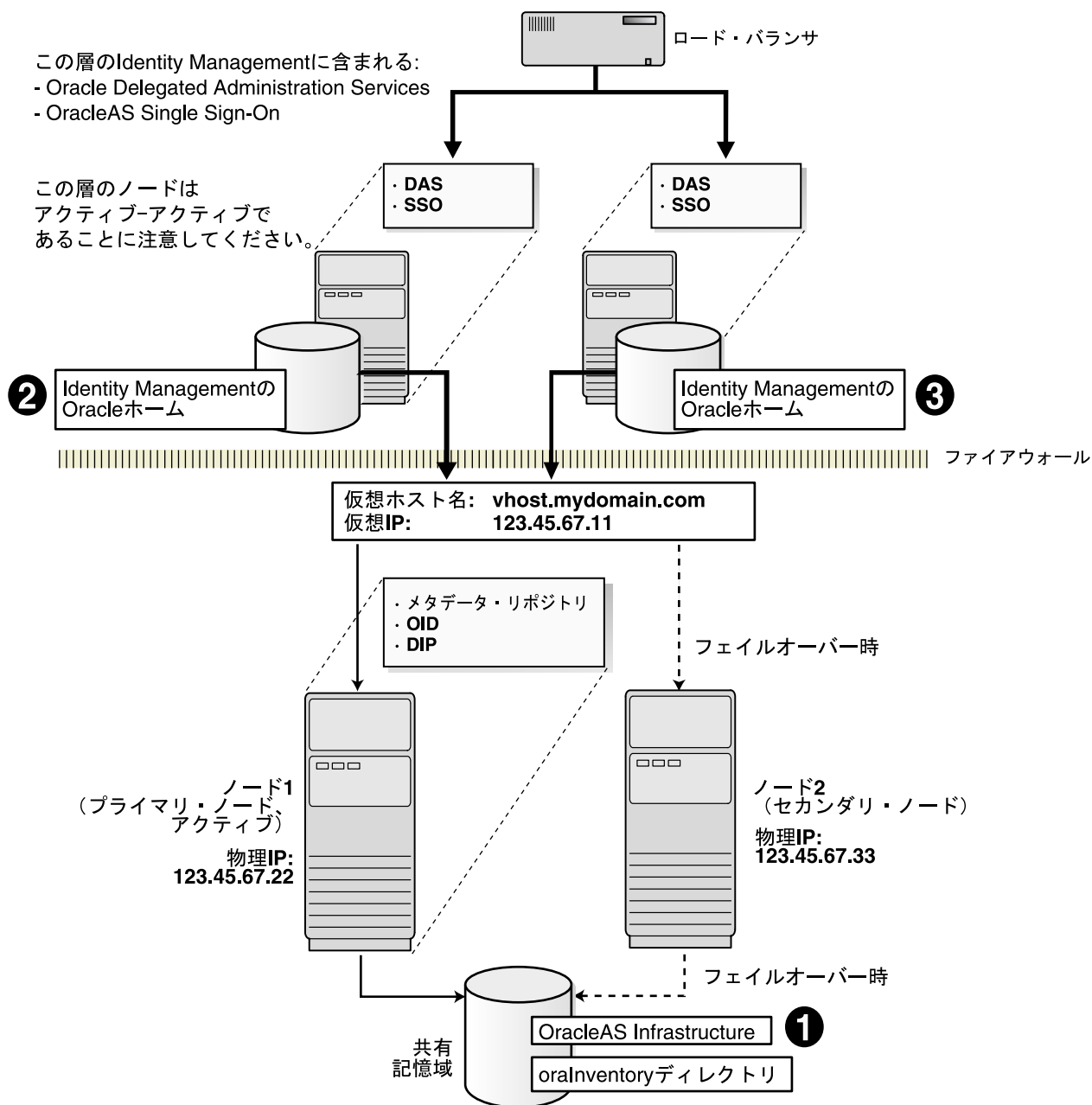
図 11-2 分散 OracleAS Cold Failover Cluster (Infrastructure) 構成
