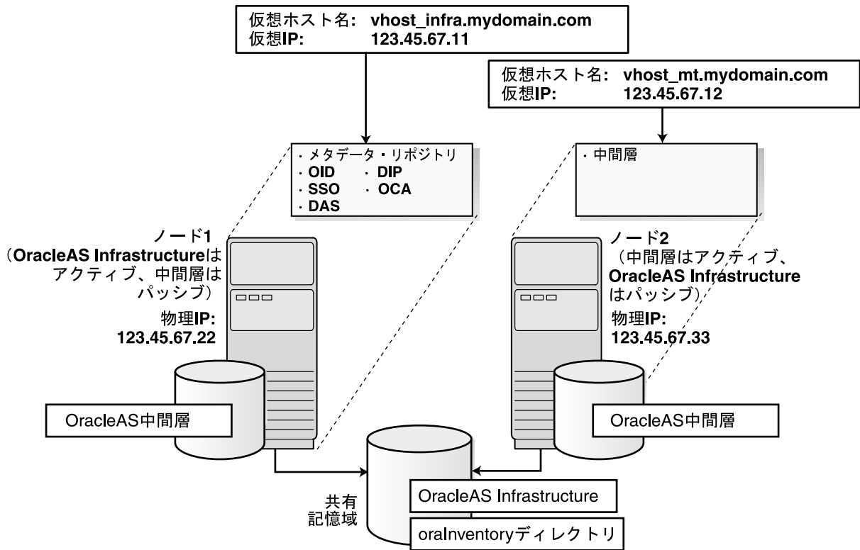
図 11-8 同じノードへの OracleAS Cold Failover Cluster (Infrastructure) および OracleAS Cold Failover Cluster (中間層)
