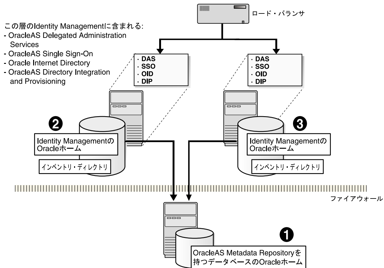
図 12-1 OracleAS Cluster (Identity Management) 構成
