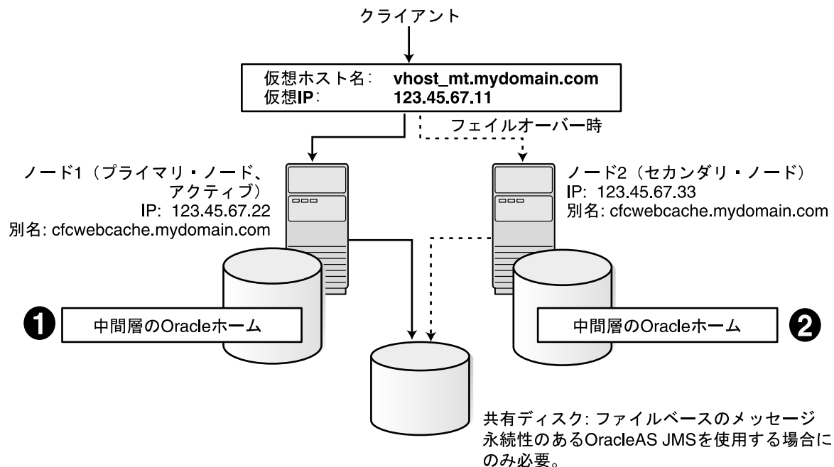
図 11-6 個別の Oracle ホームでの OracleAS Cold Failover Cluster（中間層）構成
