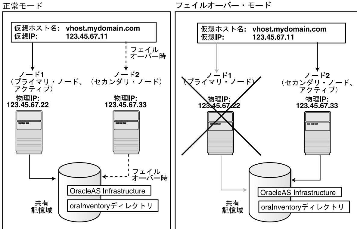
図 11-1 OracleAS Cold Failover Cluster (Infrastructure) 構成
