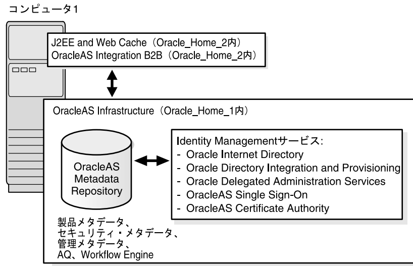
図 15-4 Integration B2B トポロジ
