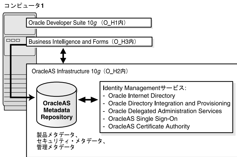
図 15-3 Forms、Reports および Discoverer アプリケーションの開発トポロジ
