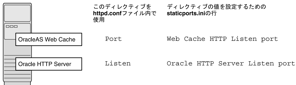
図 4-1 OracleAS Web Cache および Oracle HTTP Server の構成
