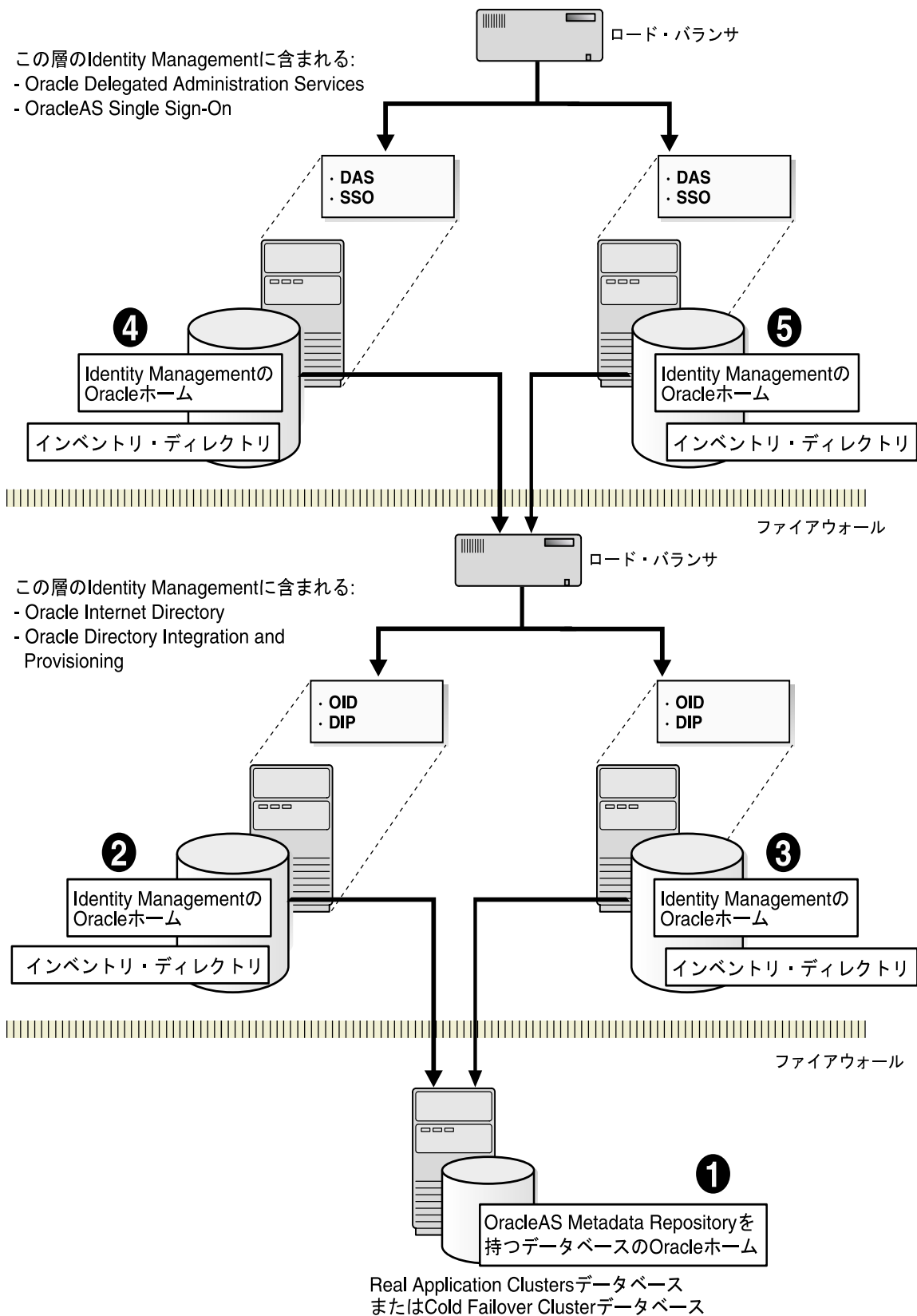
図 12-2 分散 OracleAS Cluster (Identity Management) 構成
