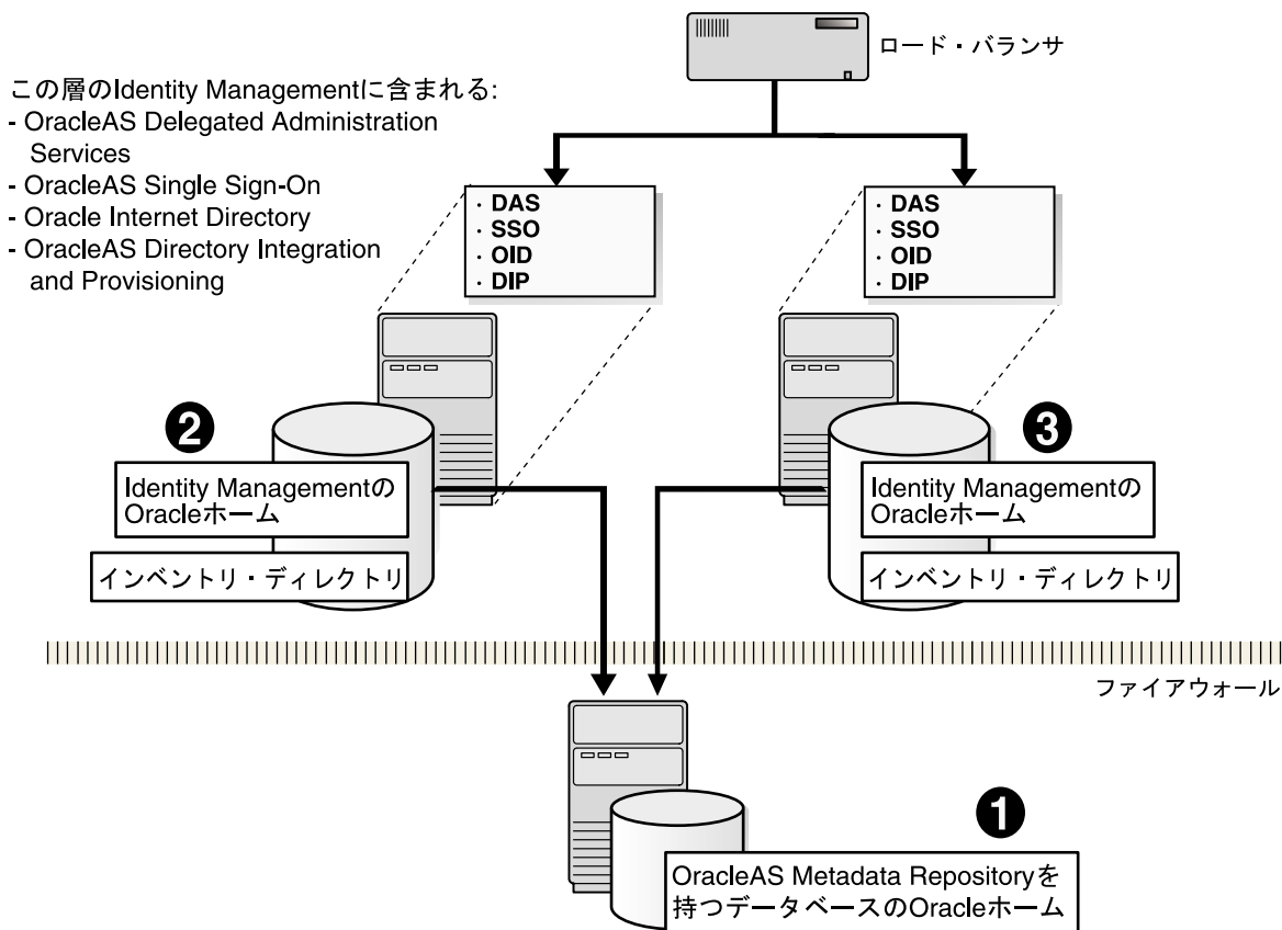
図 12-1 OracleAS Cluster (Identity Management) 構成
