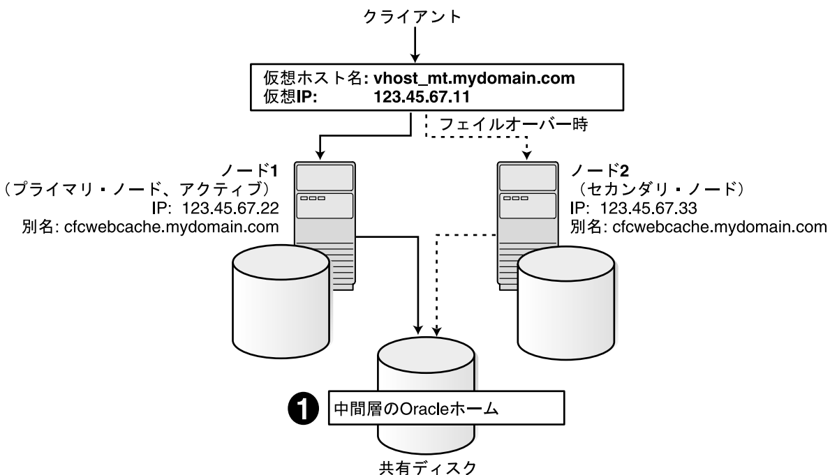
図 11-7 1 つの Oracle ホームを使用した OracleAS Cold Failover Cluster (中間層) の構成
