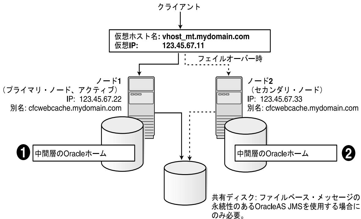
図 11-6 個別の Oracle ホームを使用した OracleAS Cold Failover Cluster (中間層) 構成
