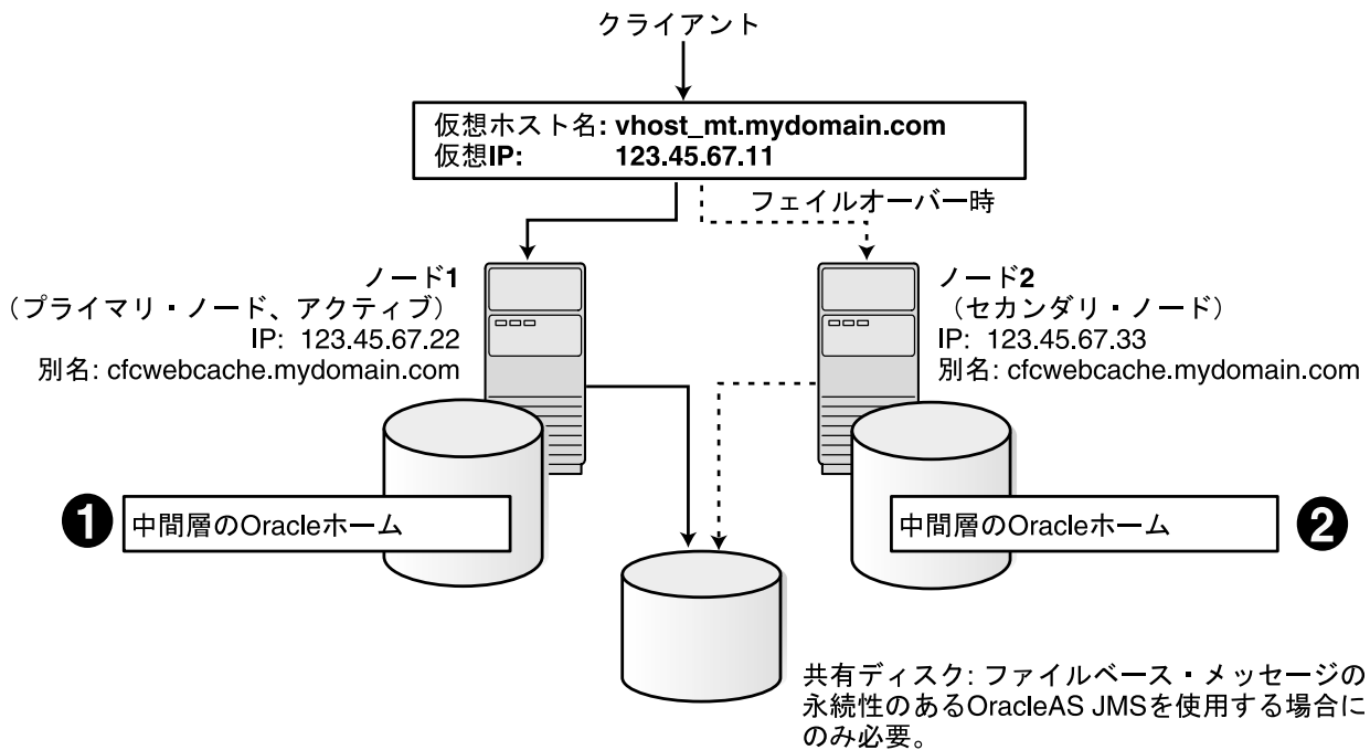
図 10-6 個別の Oracle ホームを使用した OracleAS Cold Failover Cluster (中間層) 構成
