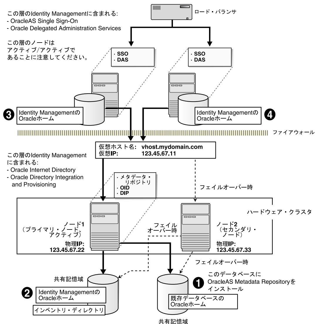
図 10-4 分散 OracleAS Cold Failover Cluster (Oracle Identity Management) 構成
