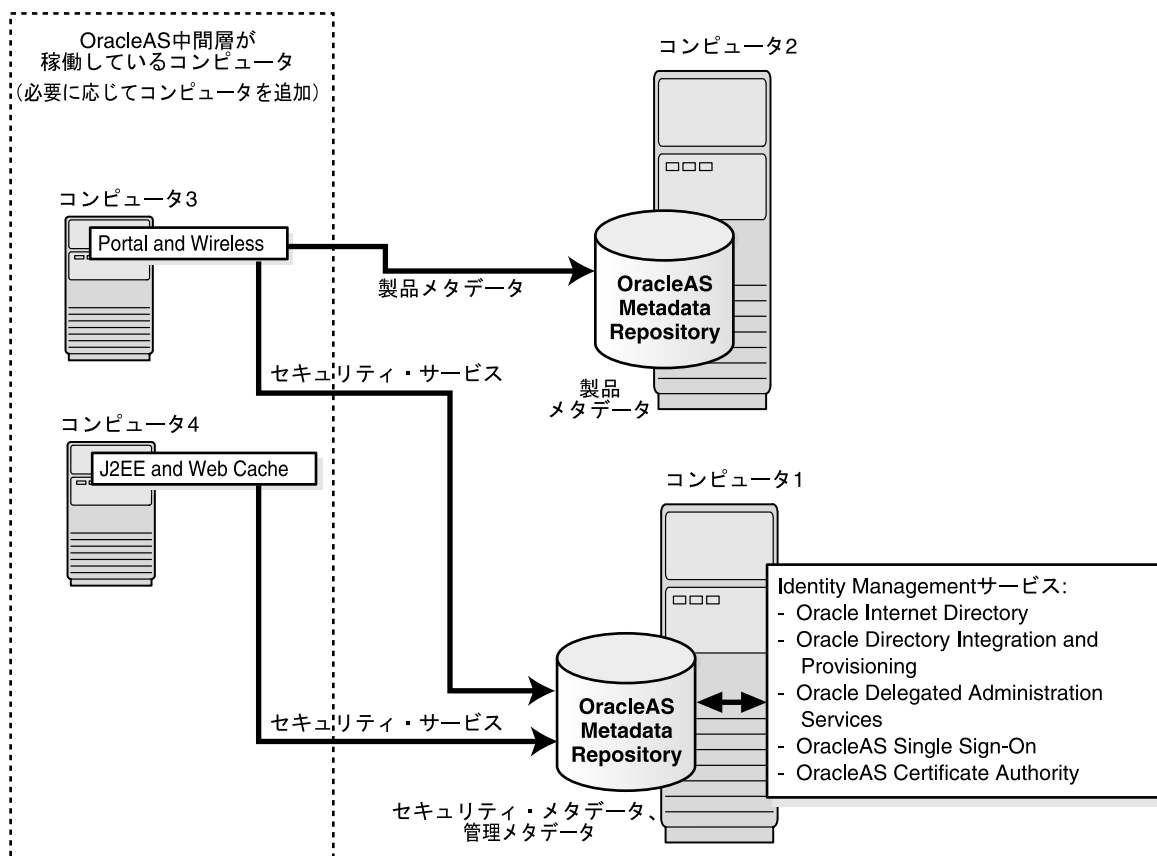
図 14-4 部門別トポロジ
