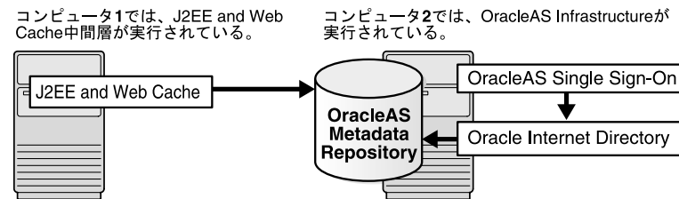
図 4-1 インフラストラクチャ・サービスを使用する中間層
