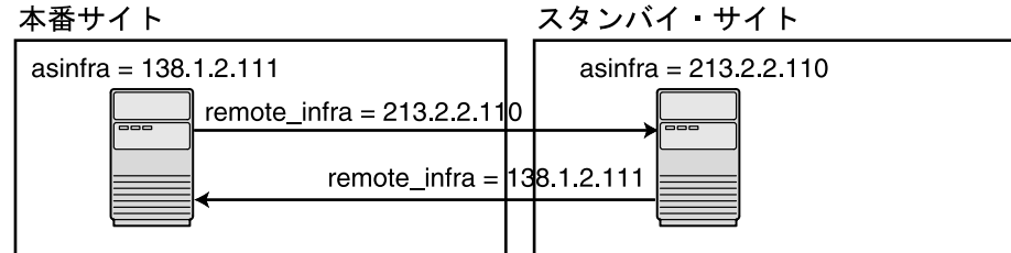
図 12-3 内部 DNS サーバー内の Oracle Data Guard エントリ
