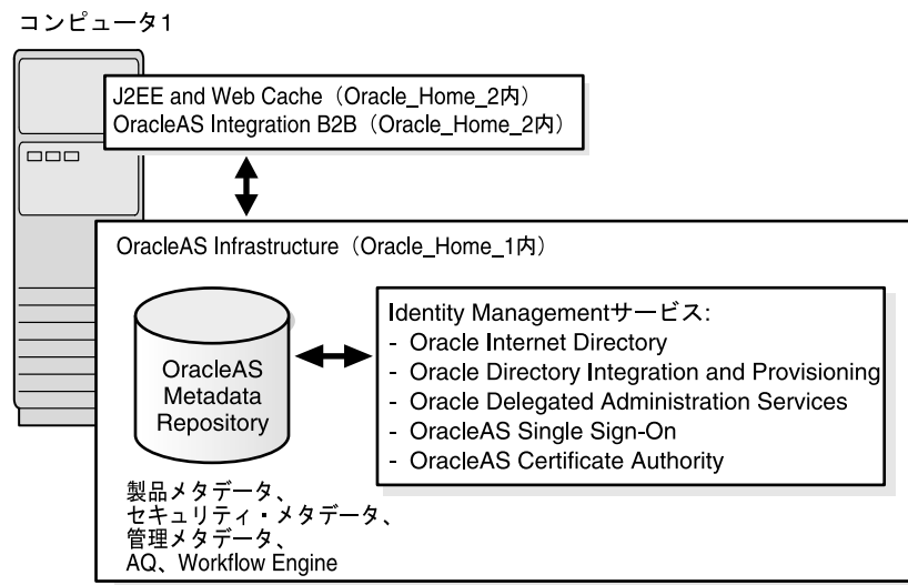
図 14-3 Integration B2B トポロジ
