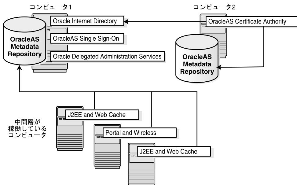
図 14-5 OCA のトポロジ
