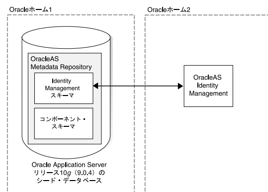
図 1-2 OracleAS Metadata Repository および OracleAS Identity Management が異なる Oracle ホームに配置された Infrastructure
