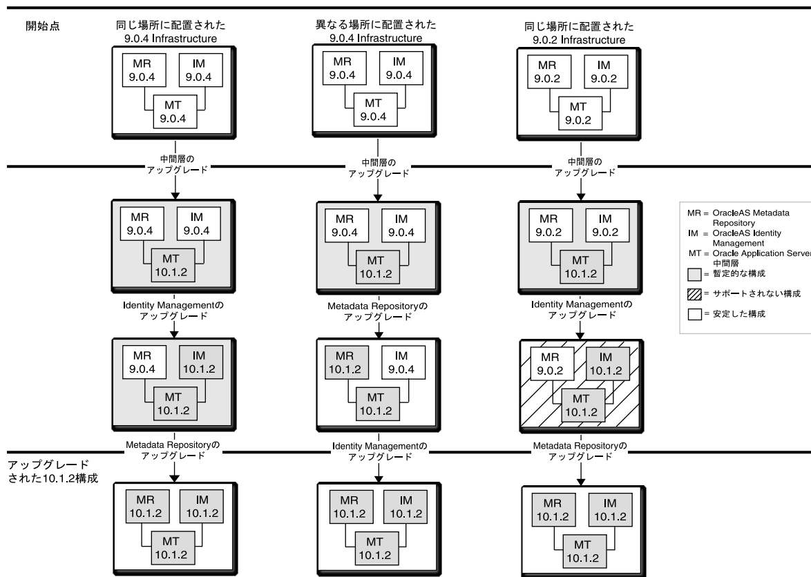
図 1-3 10g リリース 2 (10.1.2) へのアップグレード時の暫定的な構成、安定した構成およびサポートされない構成
