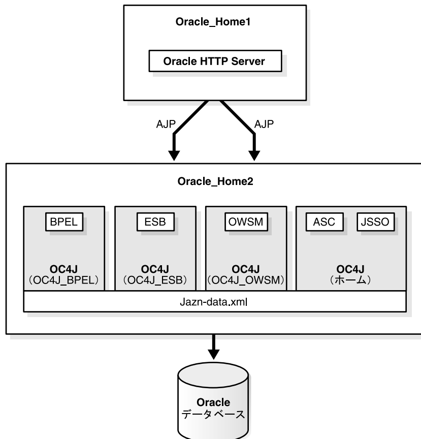
図 1-7 J2EE サーバー、個別の SOA アプリケーションおよびリモートの Oracle HTTP Server が含まれているクラスタ
