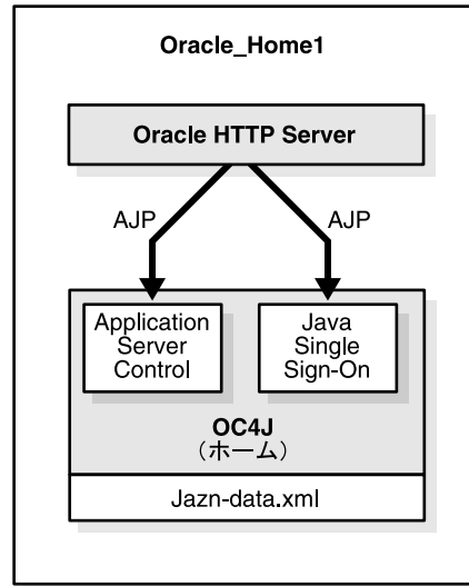
図 1-3 SOA 管理インスタンス
