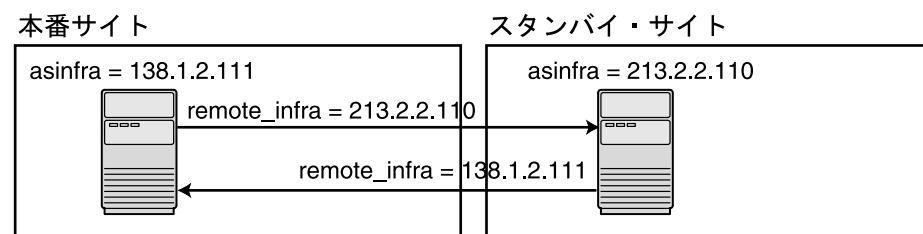
図 6-7 内部 DNS サーバー内の Oracle Data Guard エントリ
