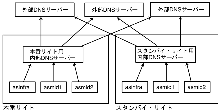
図 6-6 方法 1: DNS サーバーの使用
