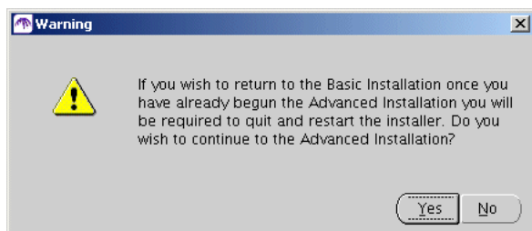
図 5-2 「警告」画面
