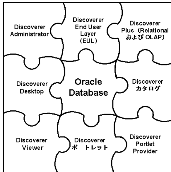
図 1-1 Oracle Discoverer のコンポーネント
