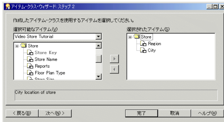
図 8-14 「アイテム・クラス・ウィザード:ステップ2」ダイアログ
