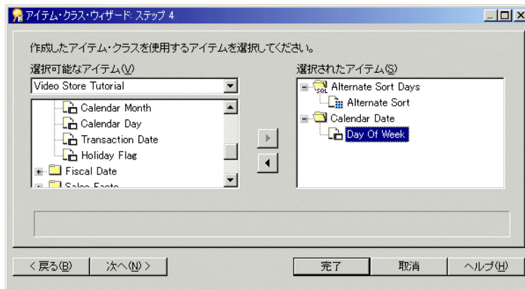
図 8-10 「アイテム・クラス・ウィザード: ステップ 4」 ダイアログ
