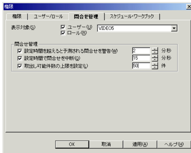
図 6-5 「権限」ダイアログ：「問合せ管理」タブ
