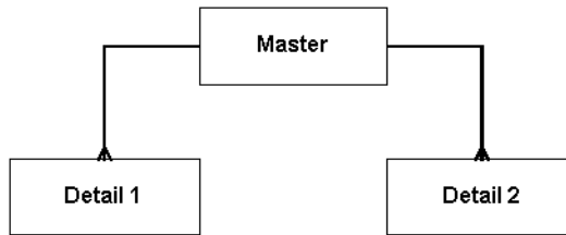
図 9-17 単純なファントラップ・スキーマ
