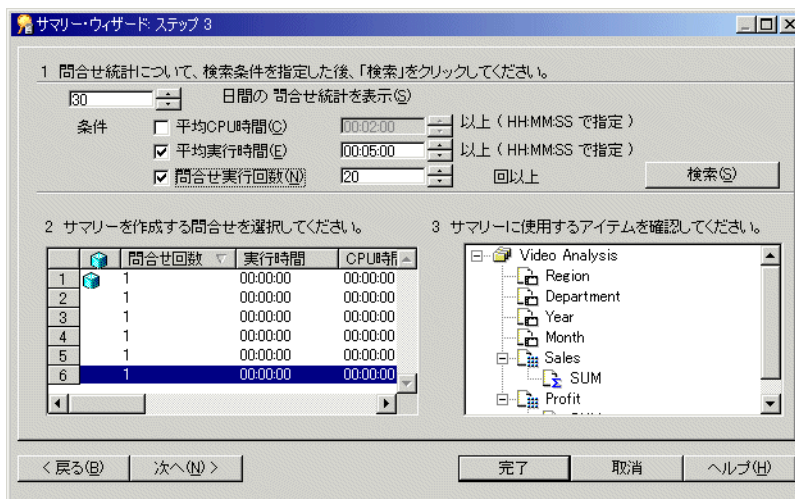
図 14-11 「サマリー・ウィザード: ステップ 3」 ダイアログ
