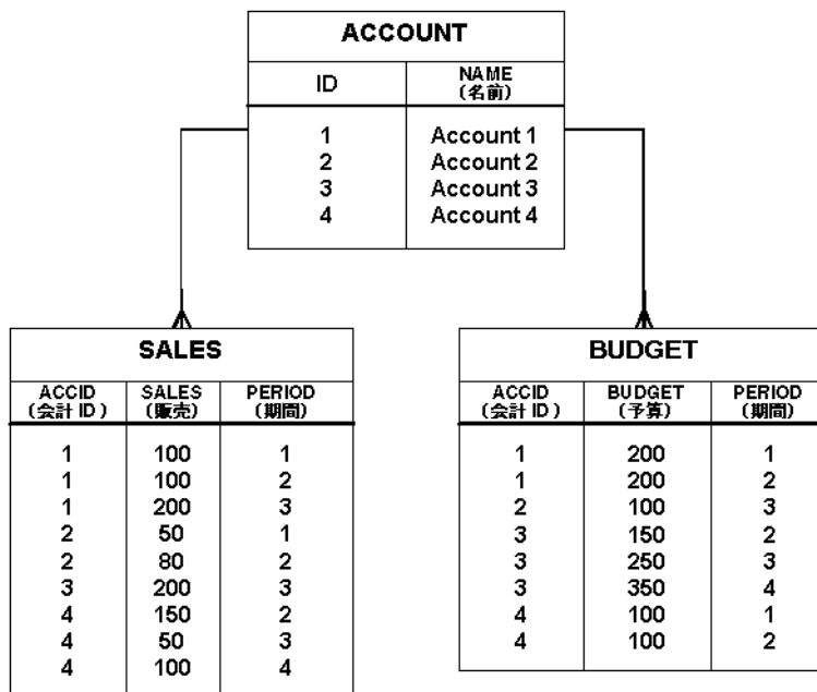
図 9-18 ファントラップ・スキーマの例
