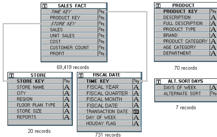
図 15-1 スキーマとデータの例
