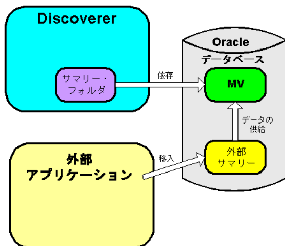
図 15-3 外部サマリーを使用する Discoverer
