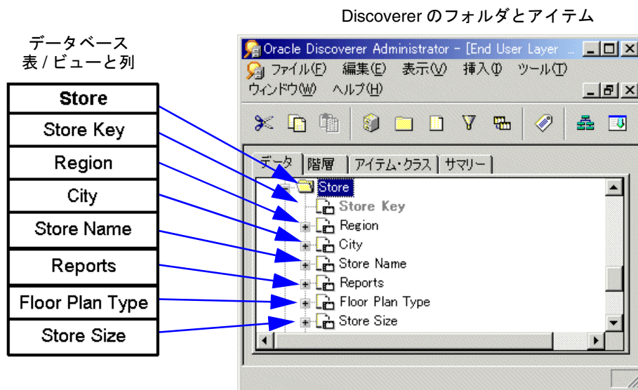
図 5-1 Discoverer Administrator による表およびビューの表現方法
