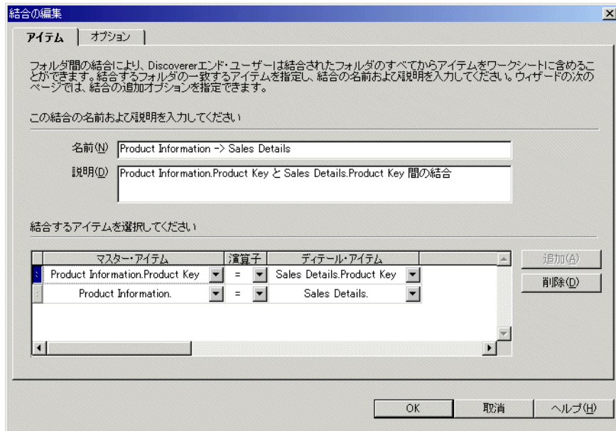
図 9-13 「結合の編集」ダイアログ:「アイテム」タブ
