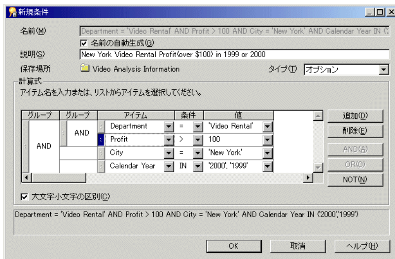
図 11-2 「新規条件」 ダイアログ (詳細設定)
