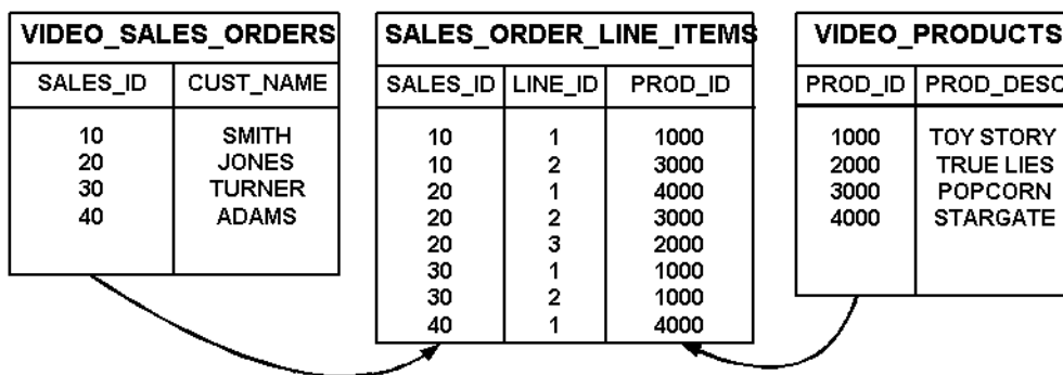
図 9-5 2 つの結合を使用して結合された 3 つの表の例
