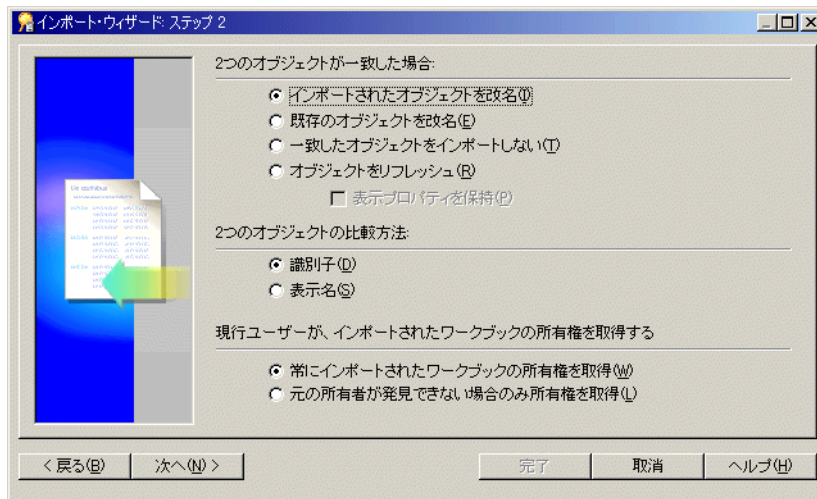
図 3-12 「インポート・ウィザード: ステップ 2」 ダイアログ
