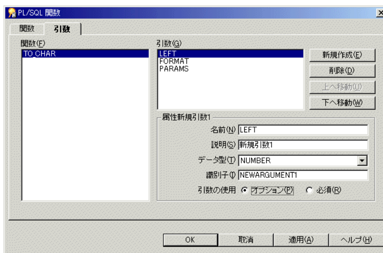
図 10-6 「PL/SQL 関数」ダイアログ: 「引数」タブ
