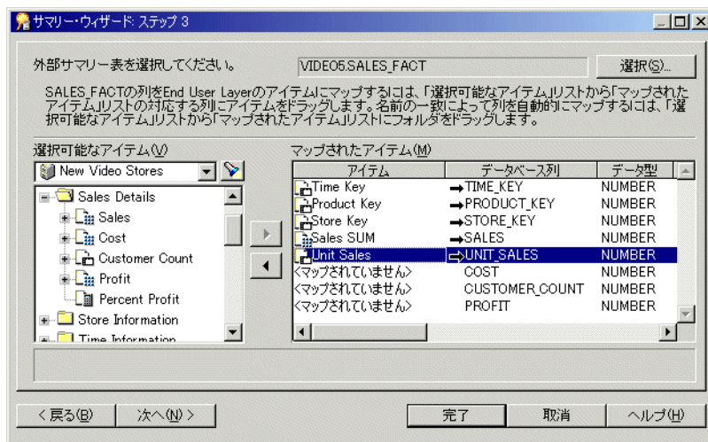
図 14-20 「サマリー・ウィザード：ステップ 3」 ダイアログ
