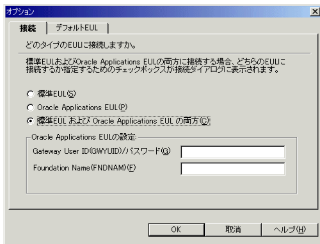
図 16-3 「オプション」ダイアログ: 「接続」タブ
