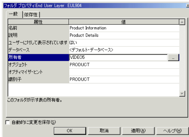
図 5-5 フォルダ・プロパティ・ダイアログ
