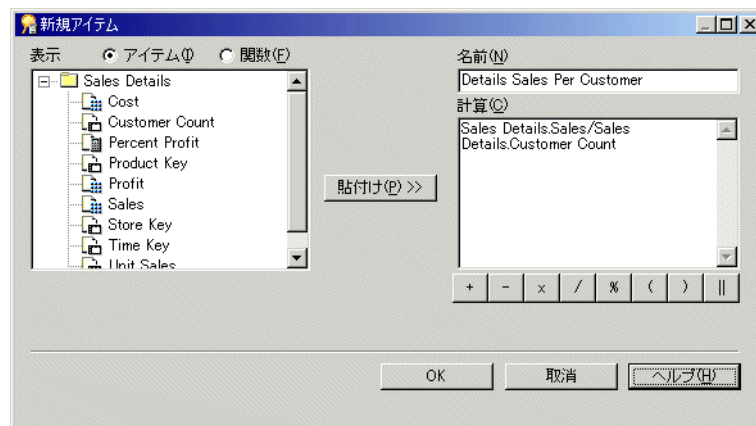
図 10-3 「新規アイテム」ダイアログ
