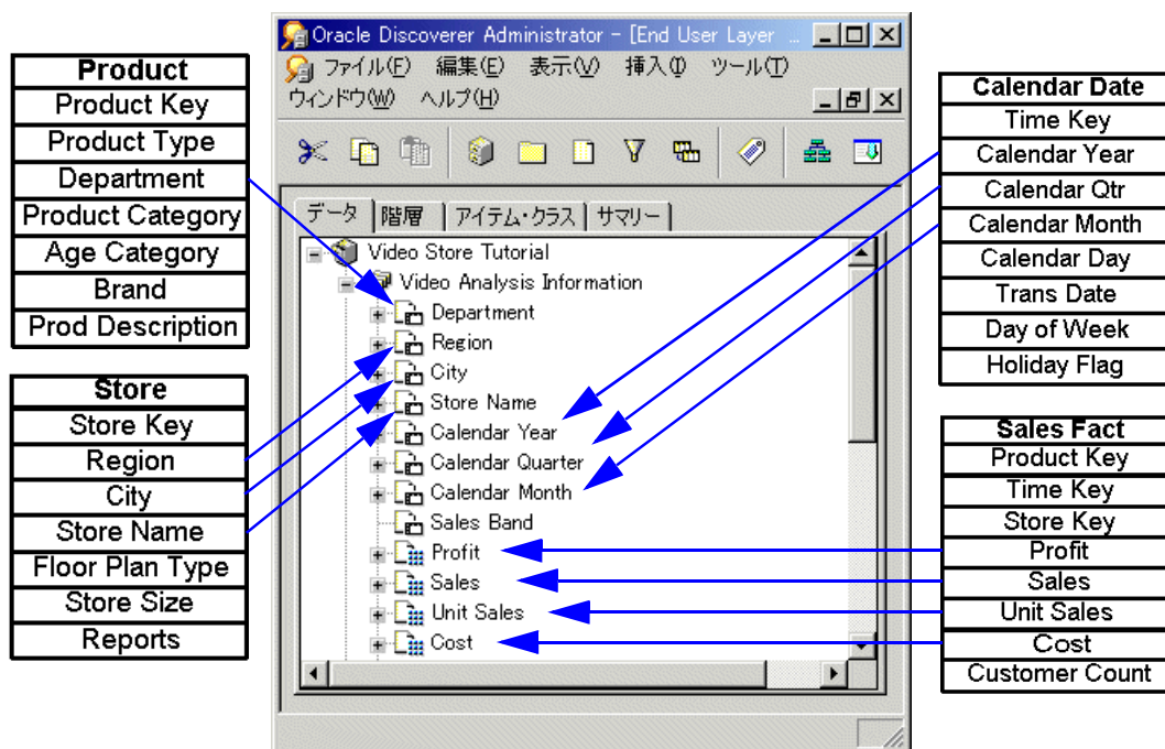
図 5-2 複合フォルダによる複数ソース表からのアイテムのグループ化方法
