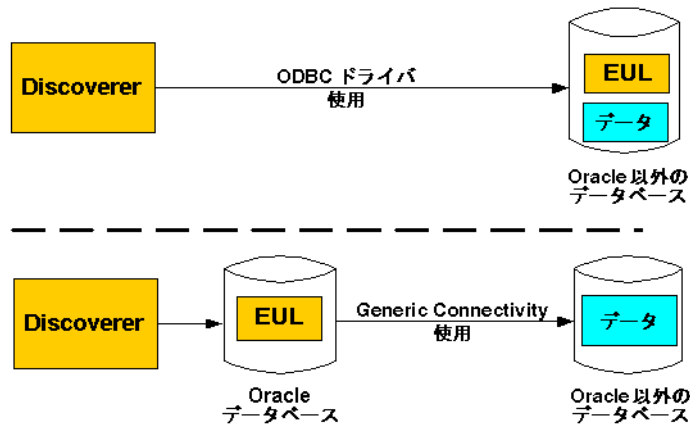
図 22-1 ODBC ドライバを使用する場合と Generic Connectivity を使用する場合の EUL の場所
