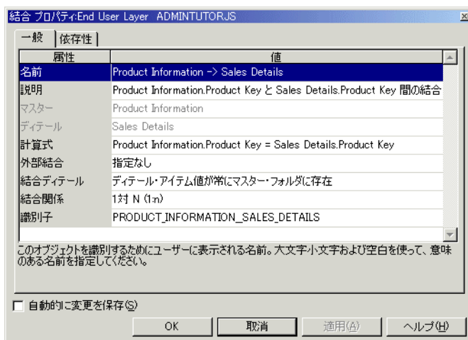
図 9-15 結合プロパティ・ダイアログ: 「一般」タブ
