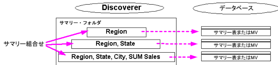
図 14-1 サマリー組合せ、サマリー・フォルダ、サマリー表またはマテリアライズド・ビューの関係
