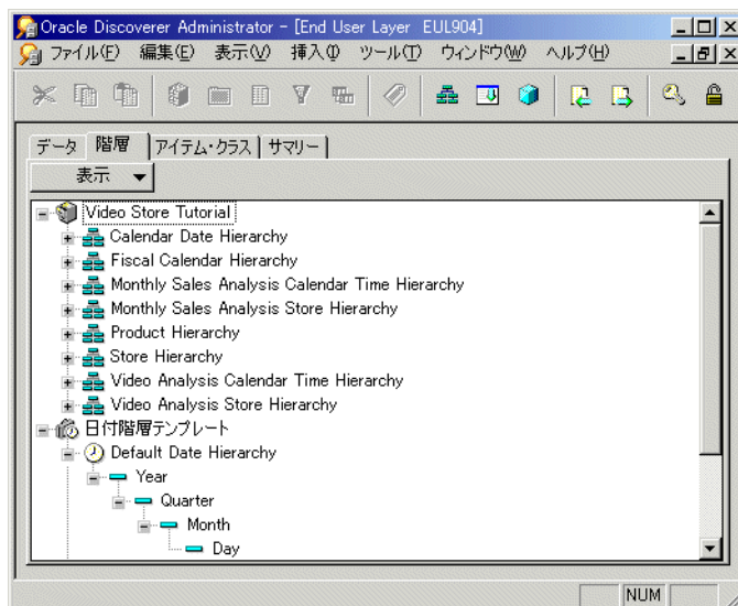
図 2-3 「ワークエリア」ウィンドウの「階層」タブ
