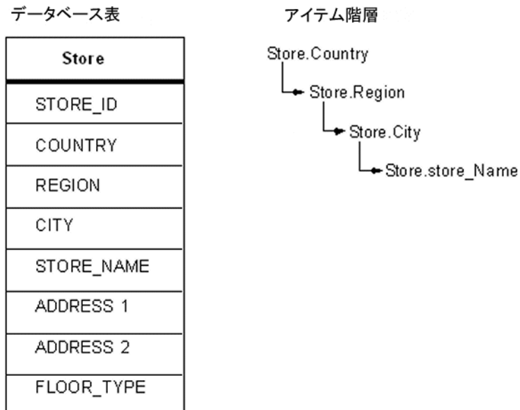
図 12-3 販売アイテム階層 – データベースの視点
