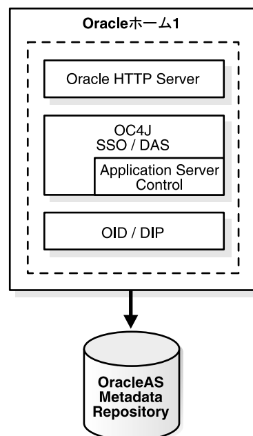
図 1-1 単一の Oracle ホームの Oracle Identity Management
