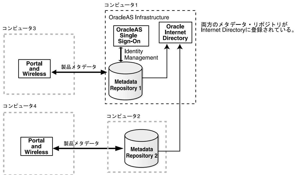
図 4-1 複数のメタデータ・リポジトリが使用されている例
