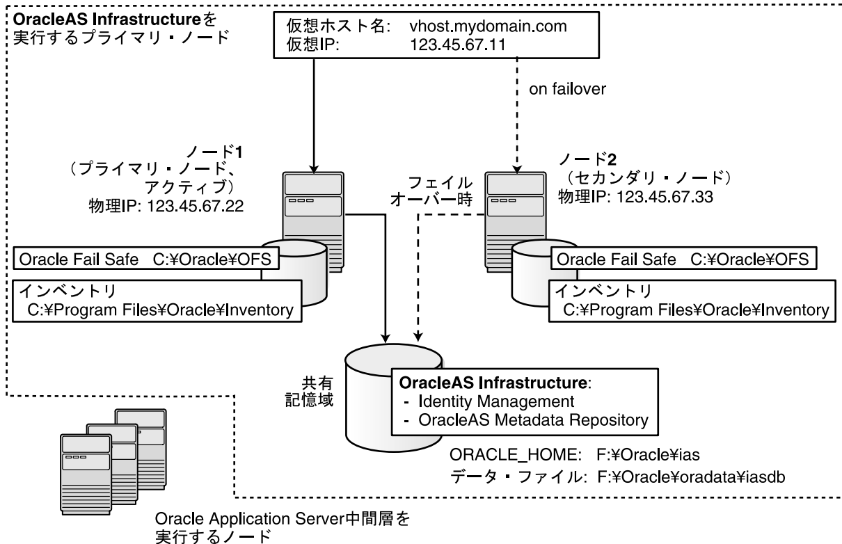
図 8-13 OracleAS Cold Failover Cluster (Infrastructure) 構成
