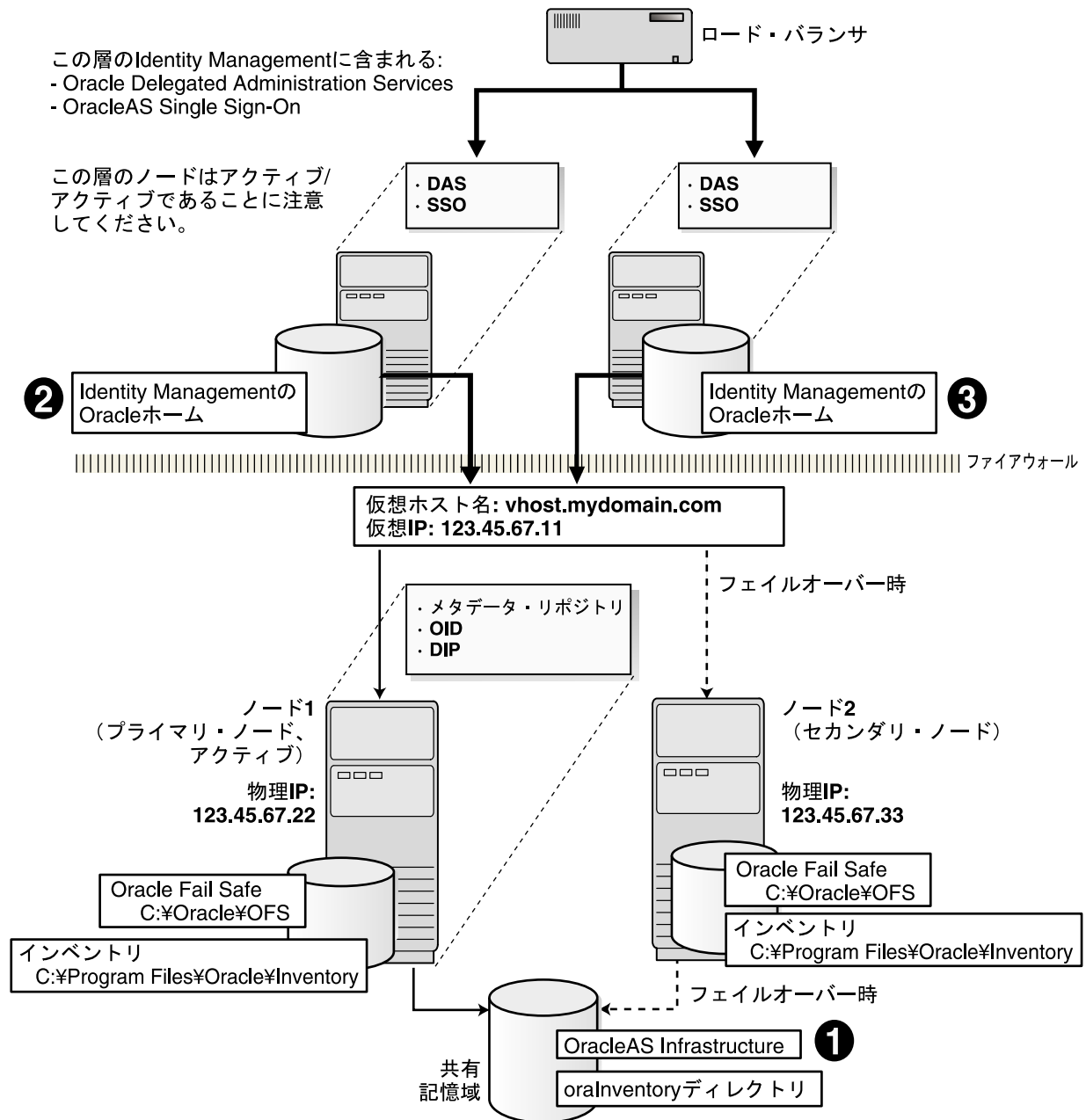
図 8-16 分散 OracleAS Cold Failover Cluster (Infrastructure) 構成
