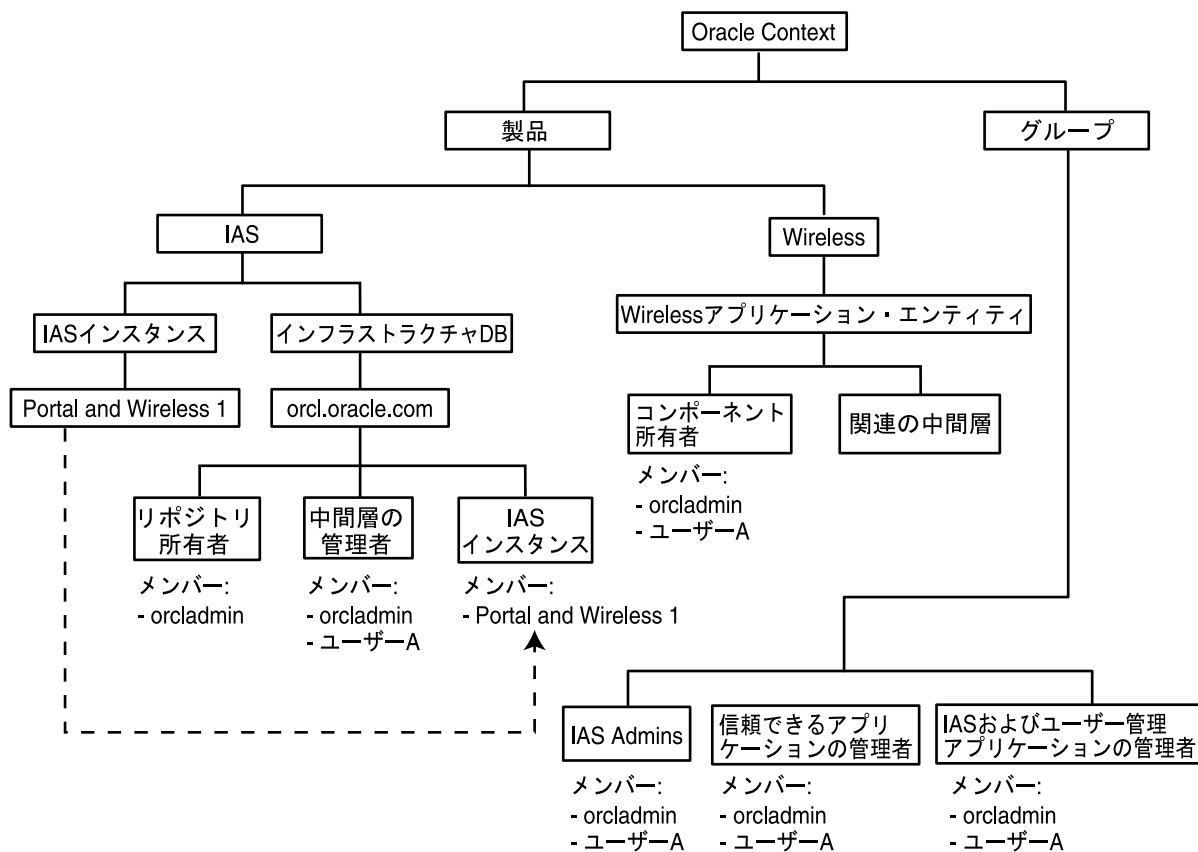
図 5-1 Infrastructure が 1 つ、中間層が 1 つある場合の Oracle Internet Directory の内容
