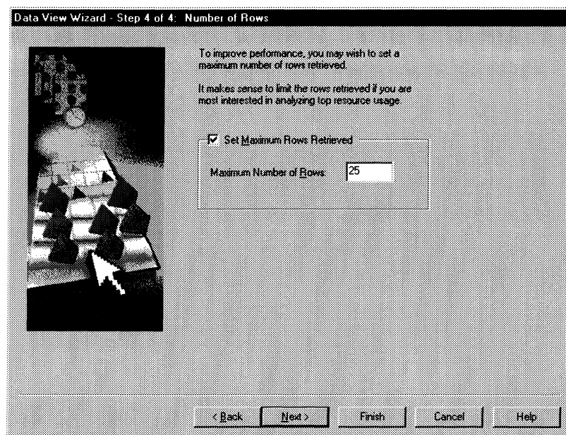
図 4-13 行数の制限
