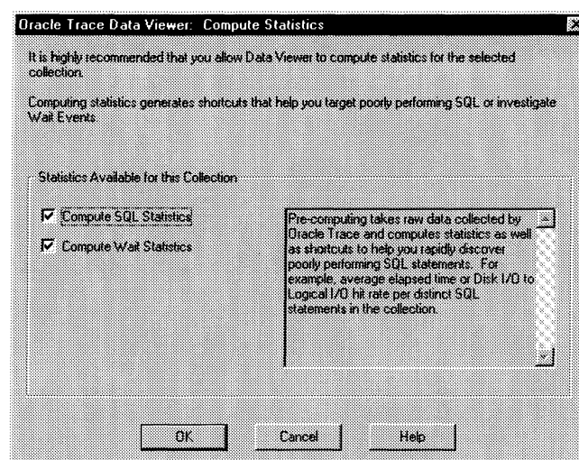
図 4-3 統計の計算
