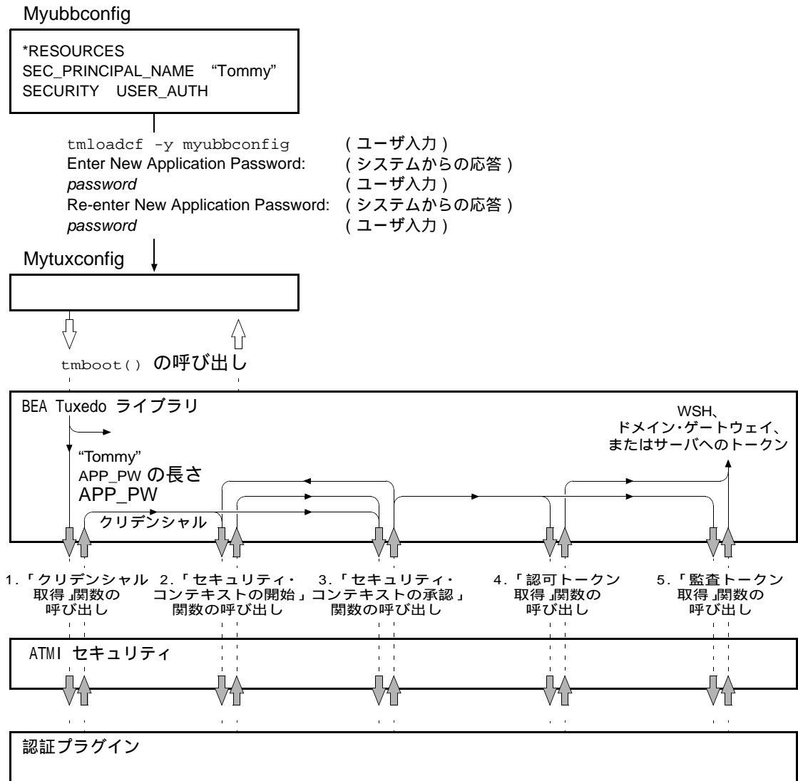
図 2-3 アプリケーションの起動時にクリデンシャルとトークンを取得する
