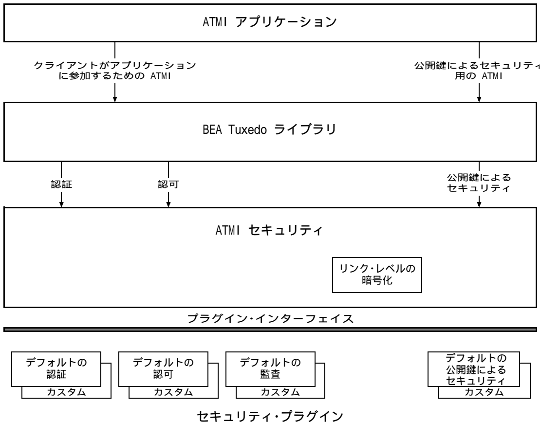
図 3-1BEA Tuxedo のセキュリティのプログラミング
