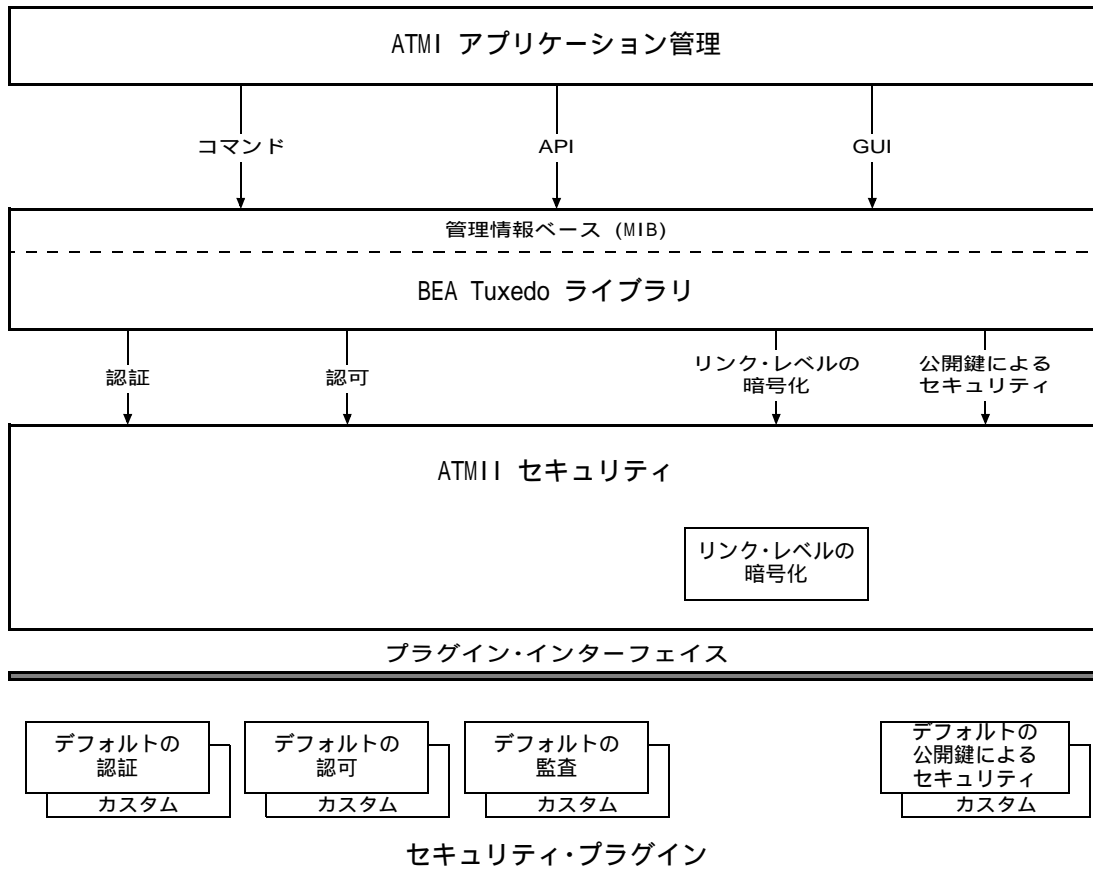
図 2-1ATMI のセキュリティの管理
