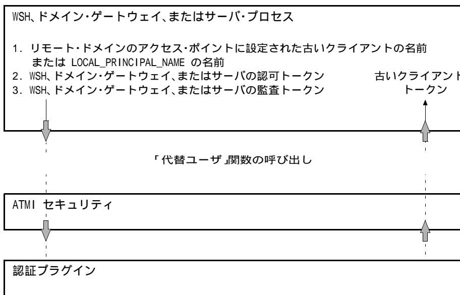
図 2-8 古いクライアントの認可トークンと監査トークンの取得
