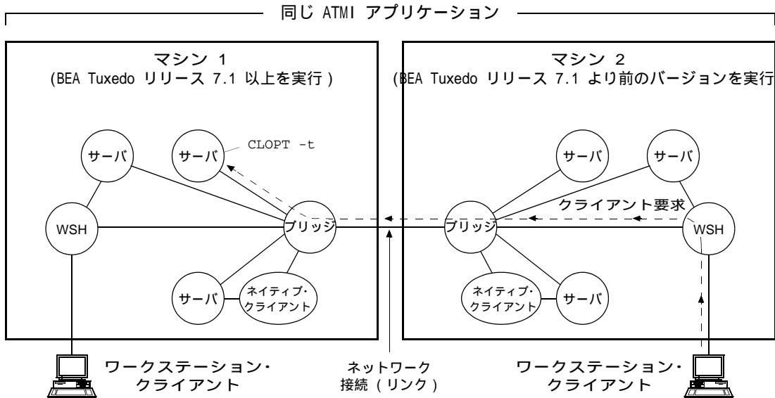
図 2-7 サーバと古い BEA Tuxedo システムの相互運用
