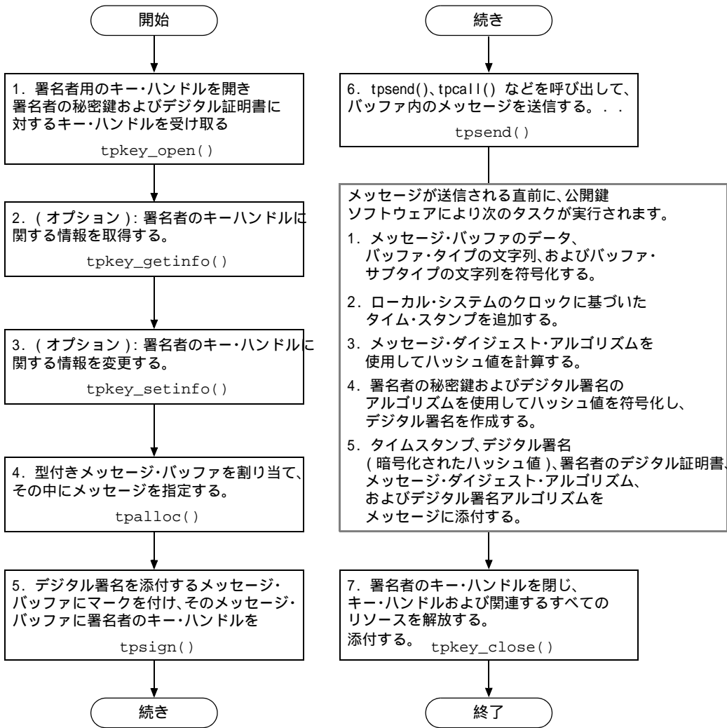
図 3-3 署名付きメッセージの送信手順
