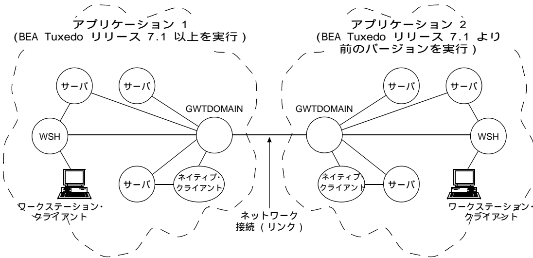
図 1-11 ドメイン間の相互運用性
