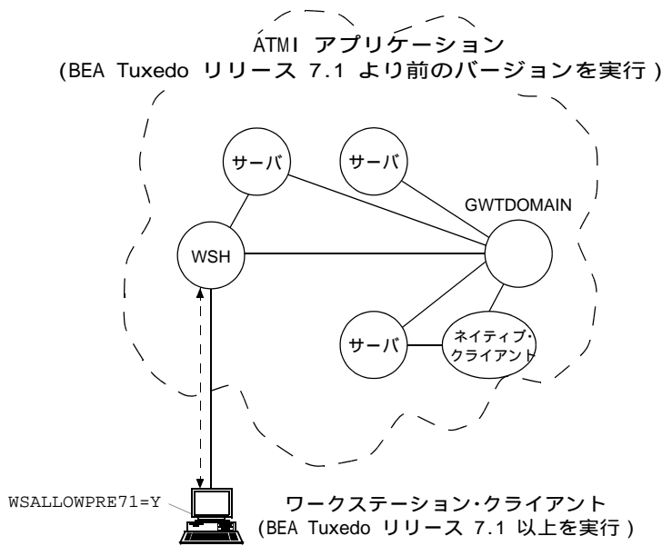
図 2-5 古い WSH と新しいワークステーション・クライアントの相互運用
