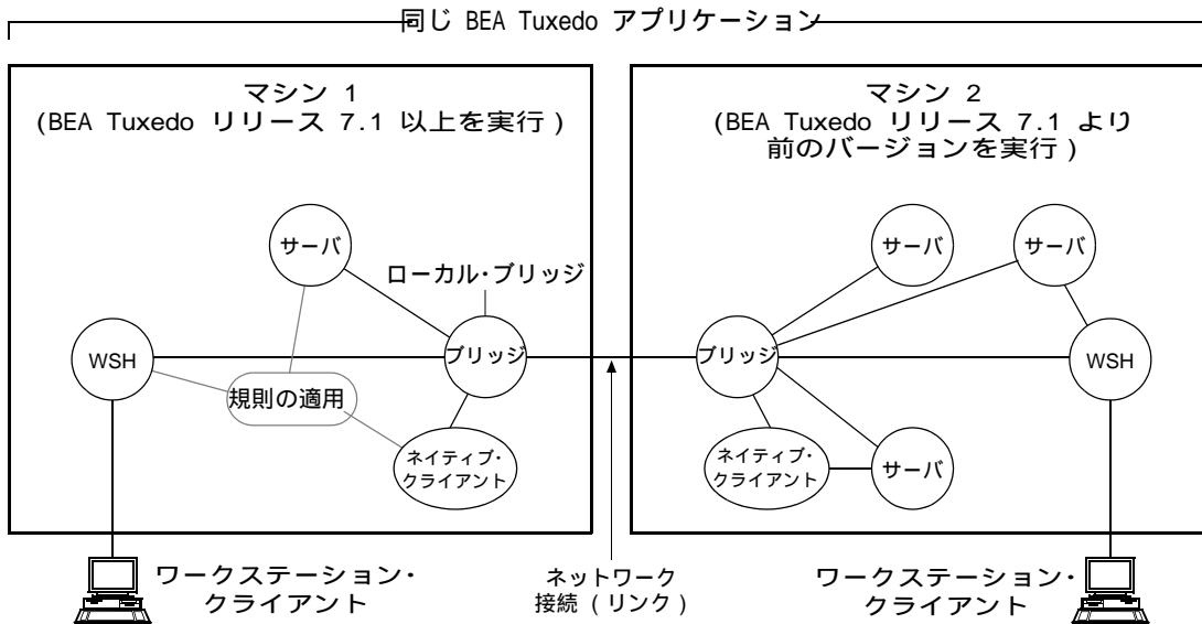
図 1-13 公開鍵によるセキュリティ機能の相互運用性規則の適用
