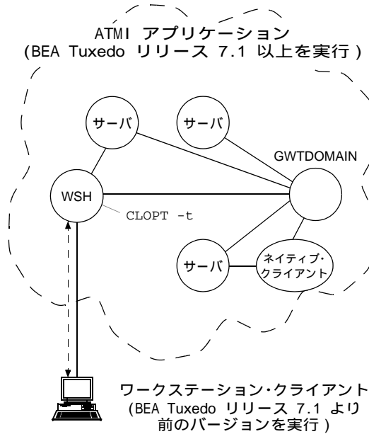
図 2-4 新しい WSH と古いワークステーション・クライアントの相互運用
