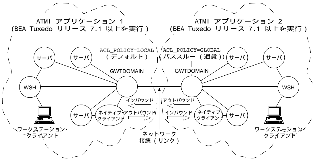
図 2-12 一方向ローカルおよび一方向グローバルの ACL 方針の確立
