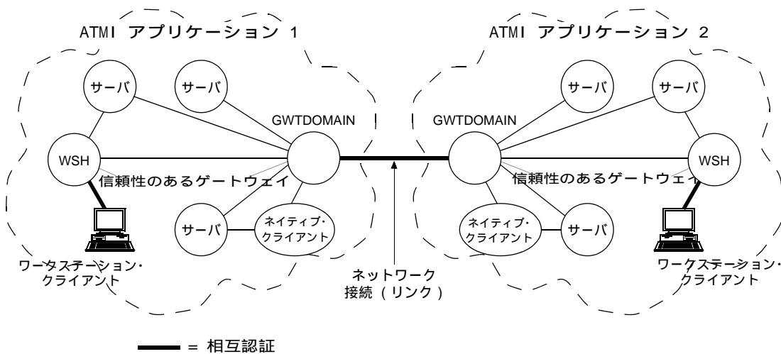
図 2-2 高信頼性委託型認証モデル
