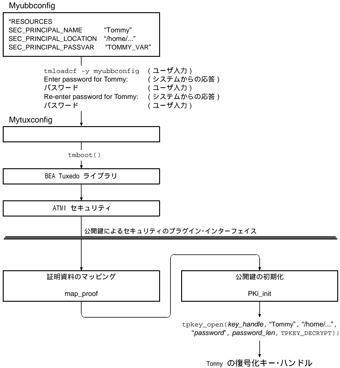
図 2-13 復号化キーの初期化例
