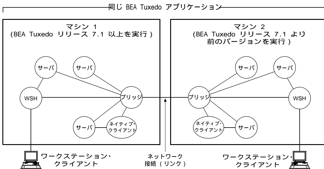
図 1-12 ドメイン内の相互運用性
