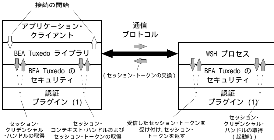
図 1-3 クライアントと WSH 間の認証
