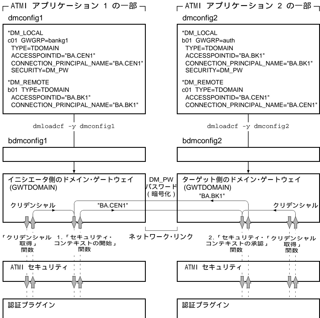
図 2-9 デフォルトの認証を使用してドメイン間にリンクを確立する
