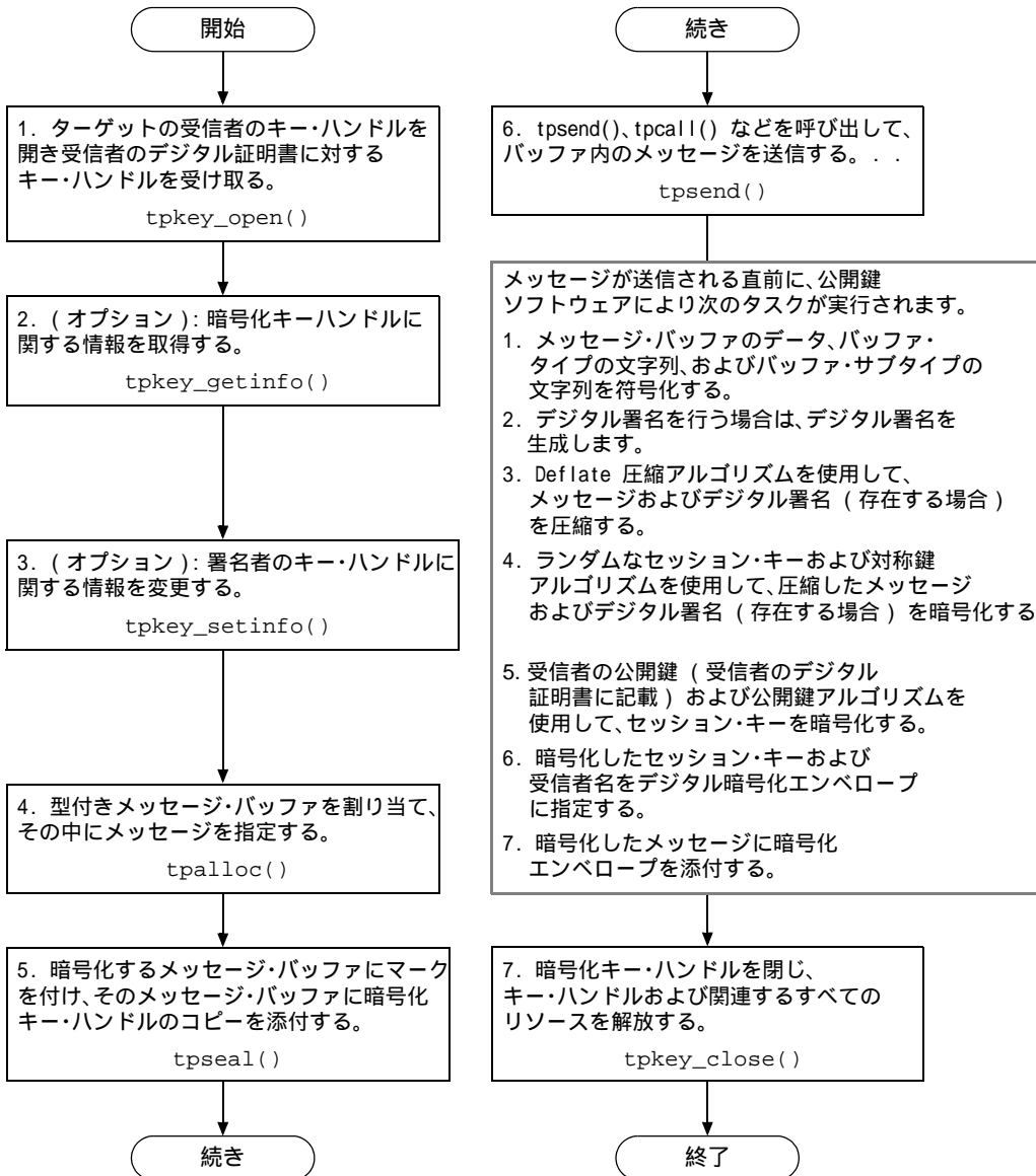
図 3-5 暗号化されたメッセージの送信手順
