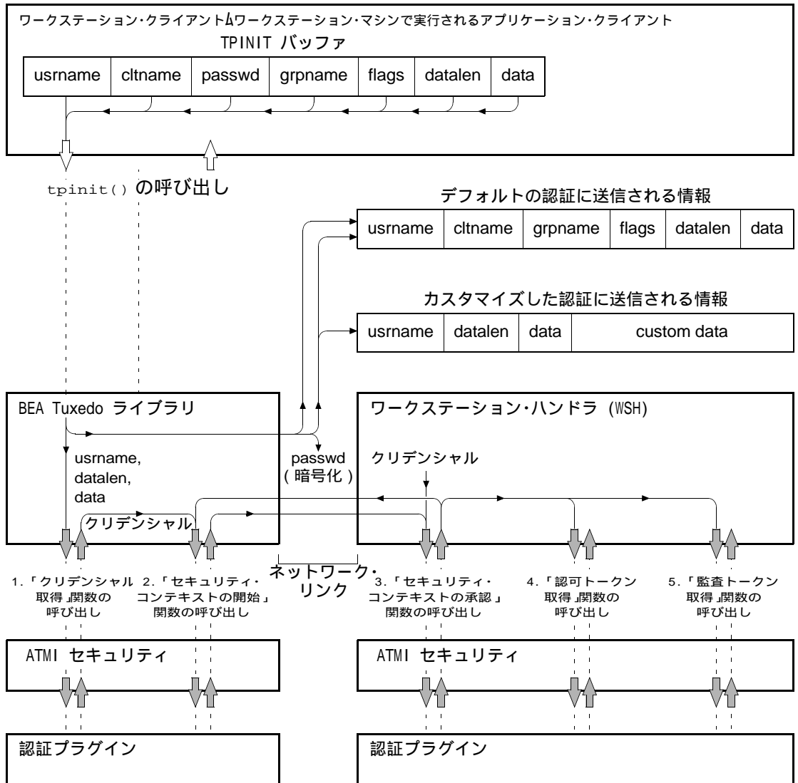
図 3-2 ワークステーション・クライアントの TPINIT バッファからデータを転送する
