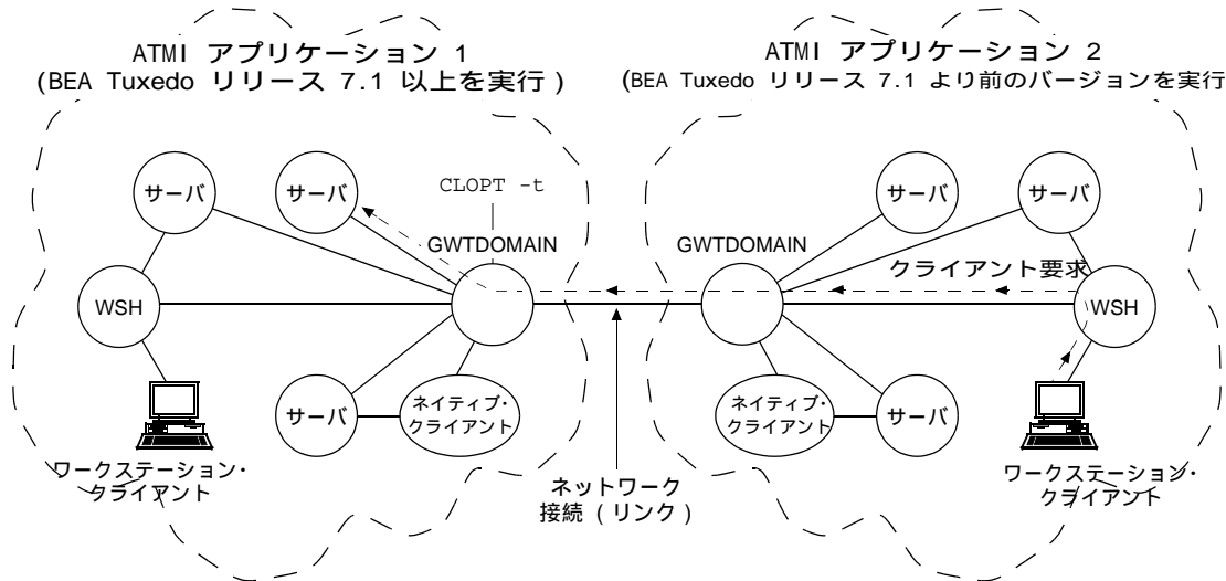
図 2-6 サーバと古い ATMI アプリケーションの相互運用
