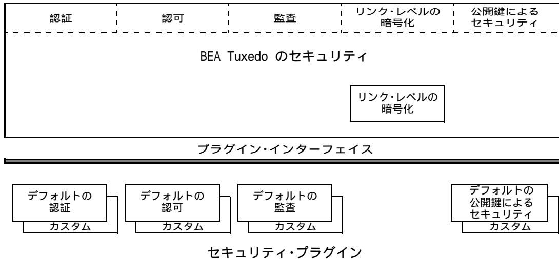
図 1-1 BEA Tuxedo ATMI プラグイン・セキュリティのアーキテクチャ
