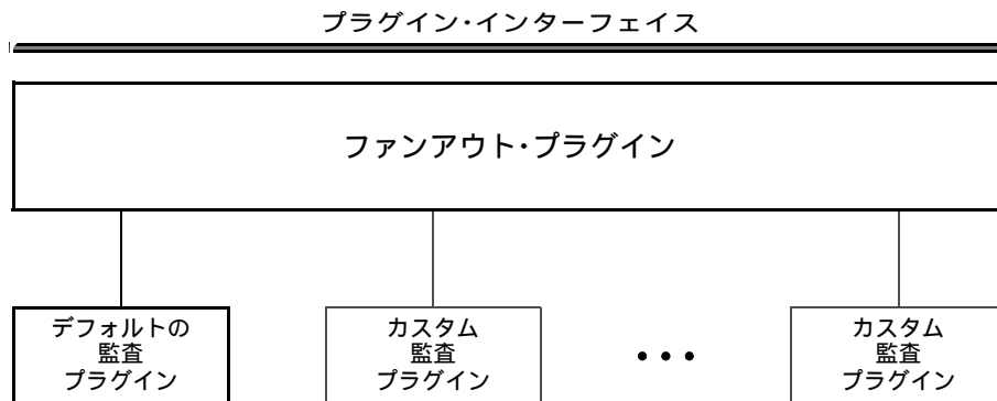
図 1-6 監査プラグインのアーキテクチャ
