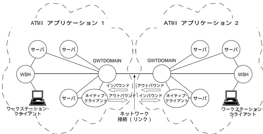
図 1-14 ATMI アプリケーション間の通信
