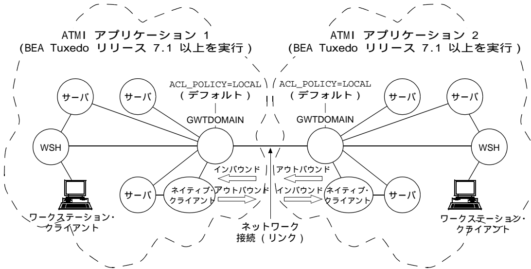
図 2-10 ローカルな ACL 方針の確立
