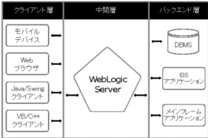
図 1-1 3層アーキテクチャ
