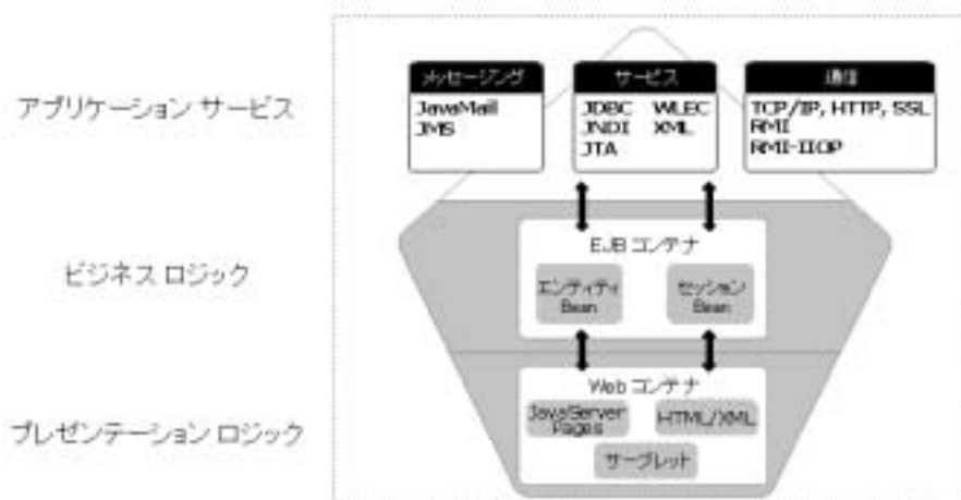
図 1-2 アプリケーションロジックのレイヤ
