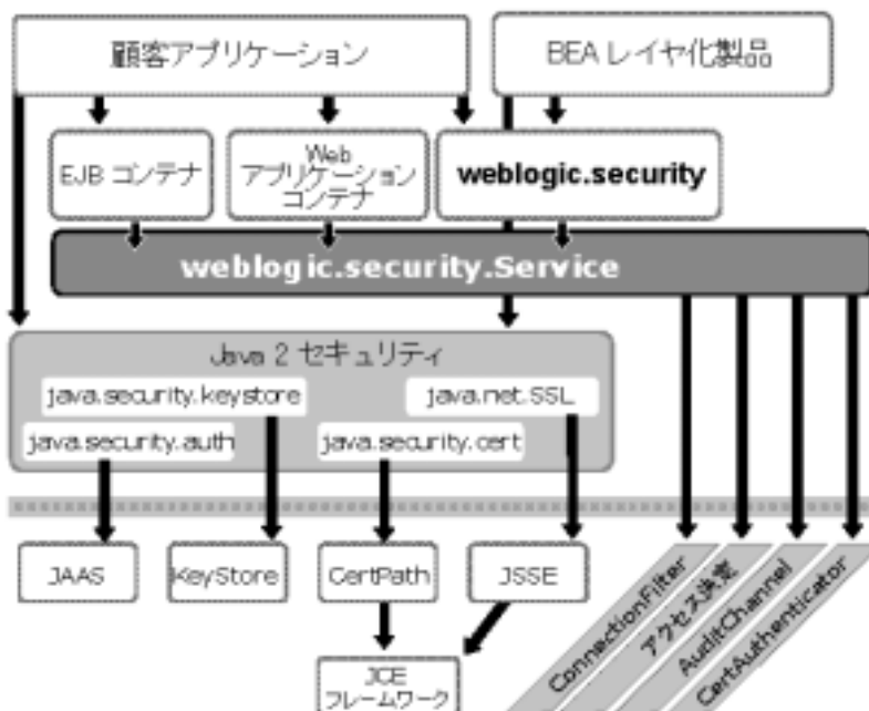
図 2-1 WebLogic セキュリティ サービス
