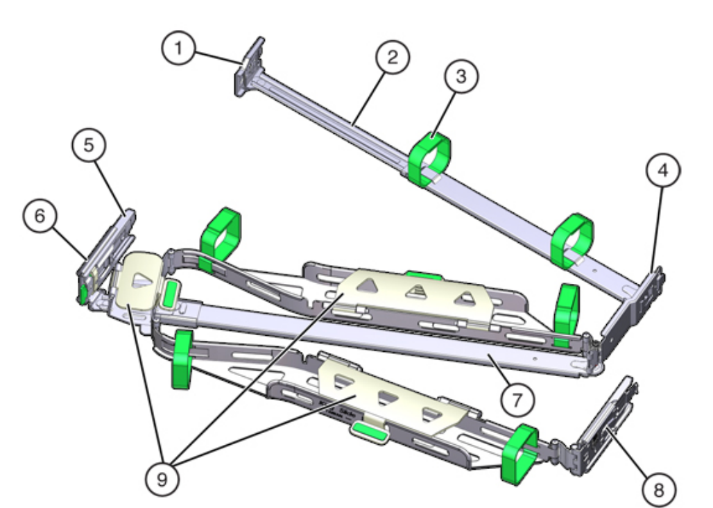
图 30 ZS5-2 控制器理线架
