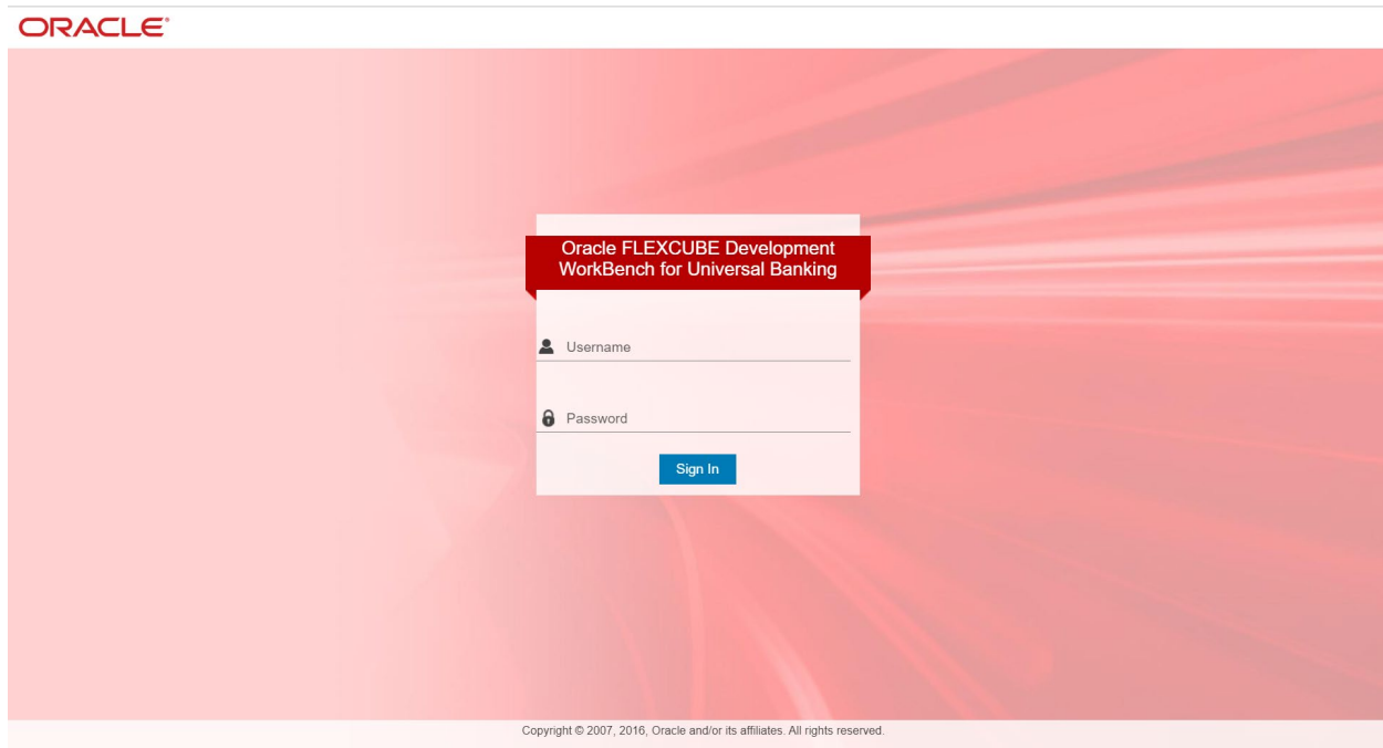
Fig 4.1 Login Page
