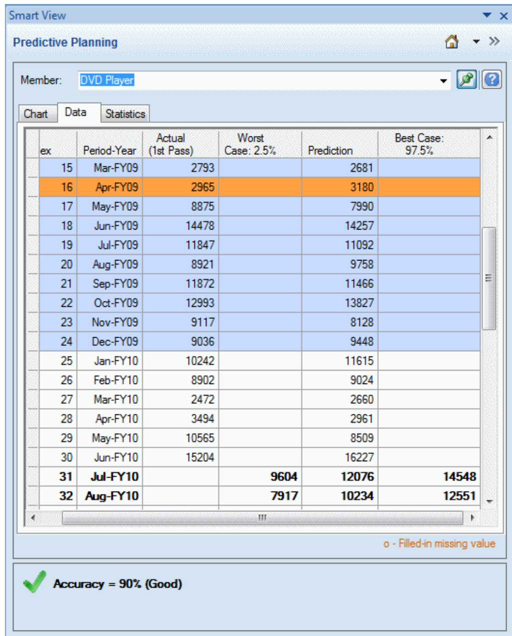
Figura 2-2 Painel do Planejamento Preditivo, Guia Dados
