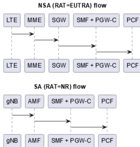
Figure 4-5 NSA and SA Flow
