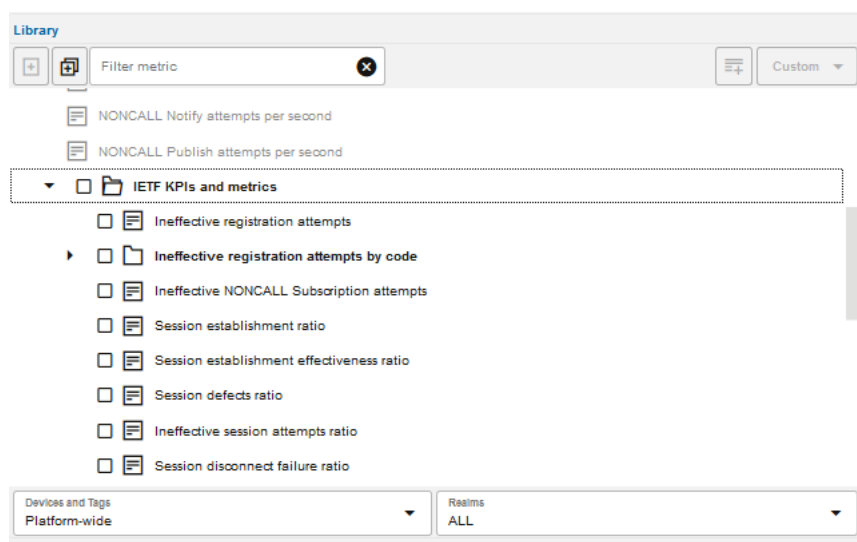
Figure 4-3 IETF KPIs
