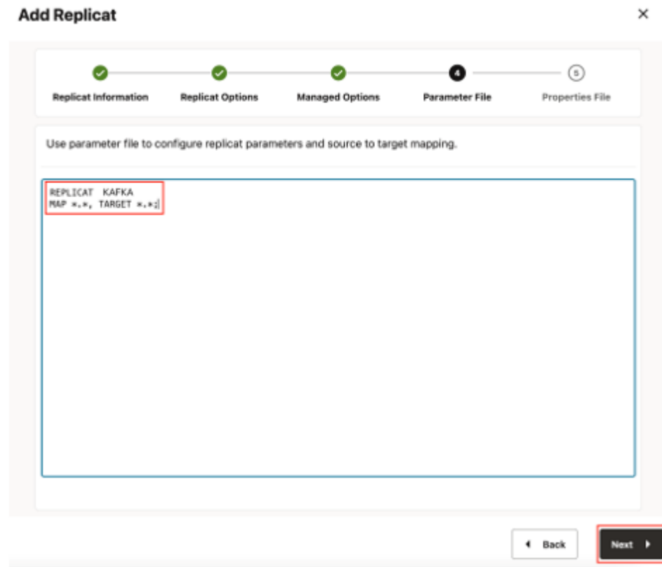
Figure 8-80 Parameter File
