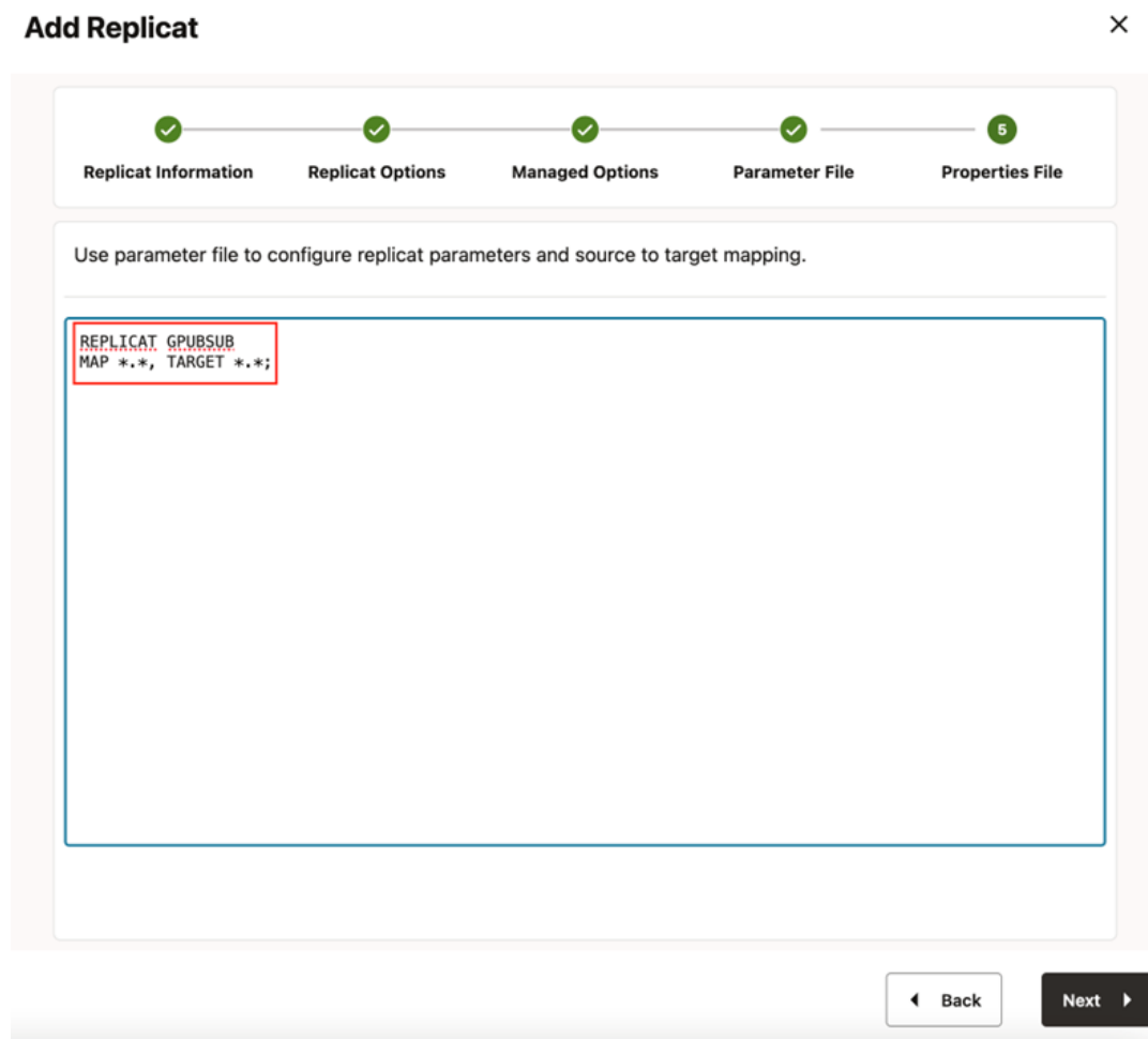
Figure 8-73 Parameter File
