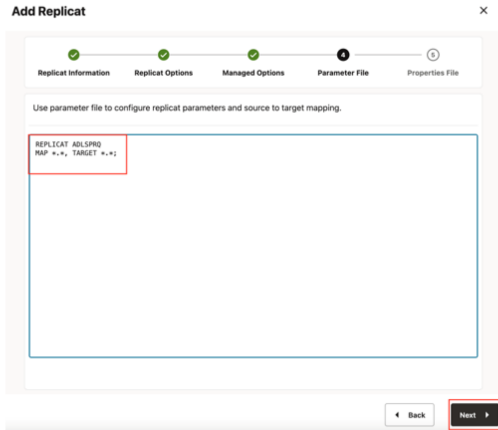
Figure 8-32 Parameter File
