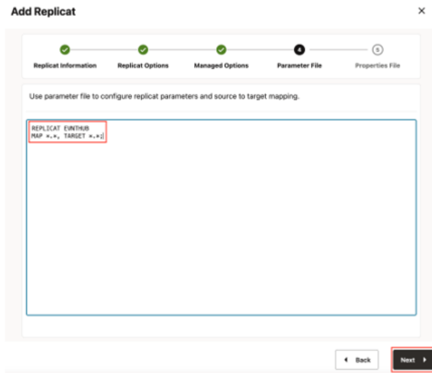
Figure 8-56 Parameter File
